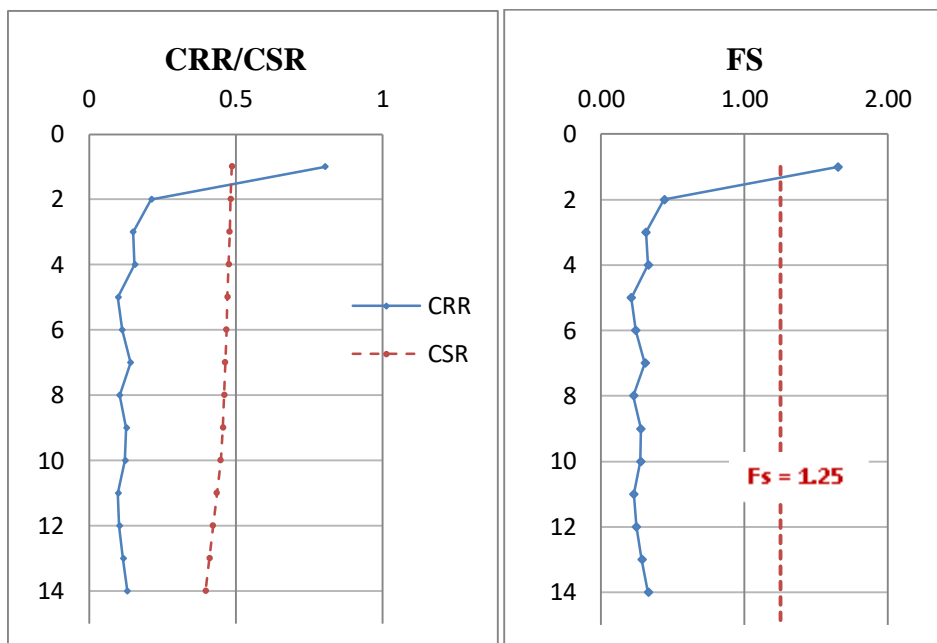
Figure 36: Variation de CRR, CSR et FS en profondeur (sondage N°03)
