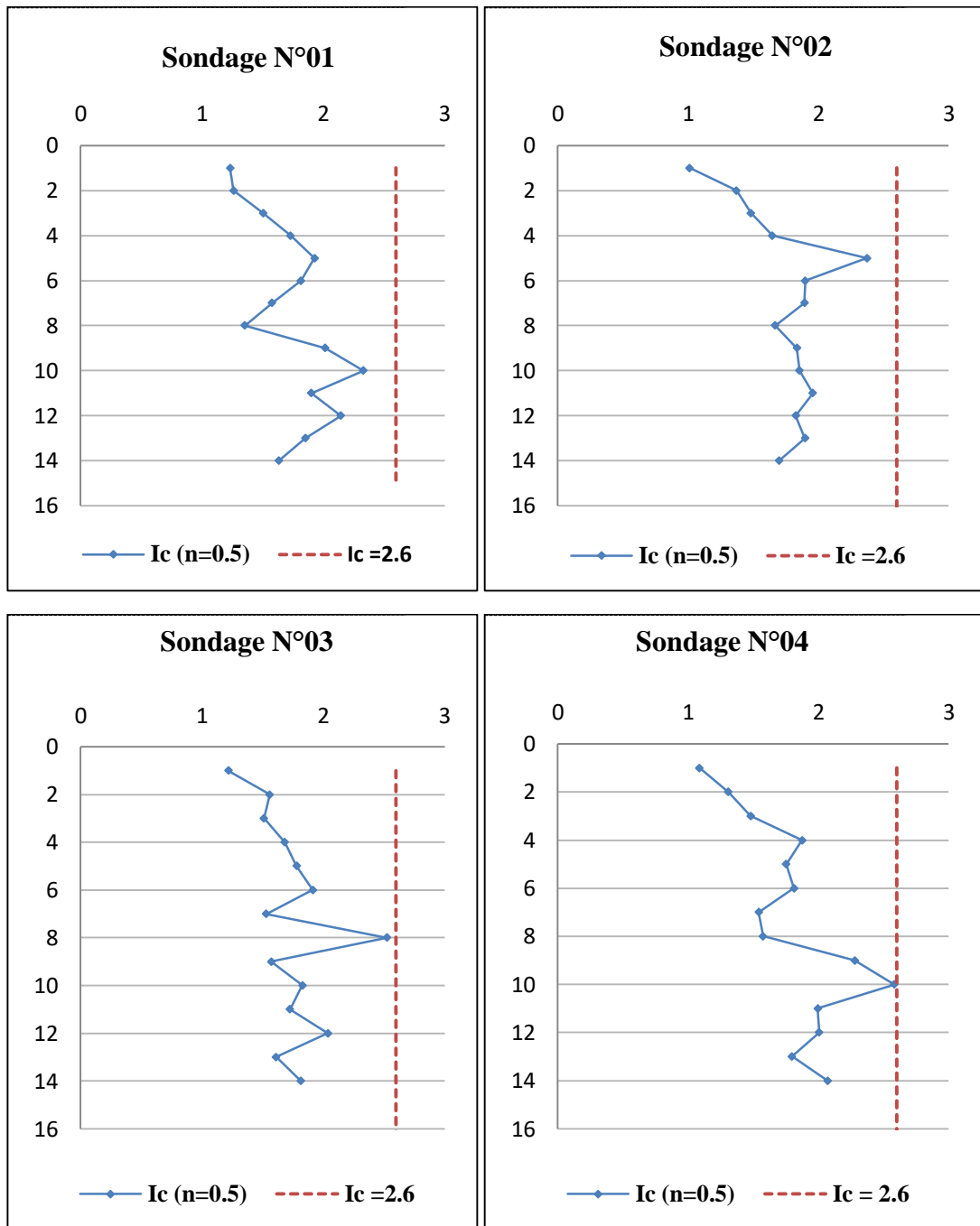
Figure 433: Profile de I_c (n=0.5) des sondages N°01, 02,03 et 04.
