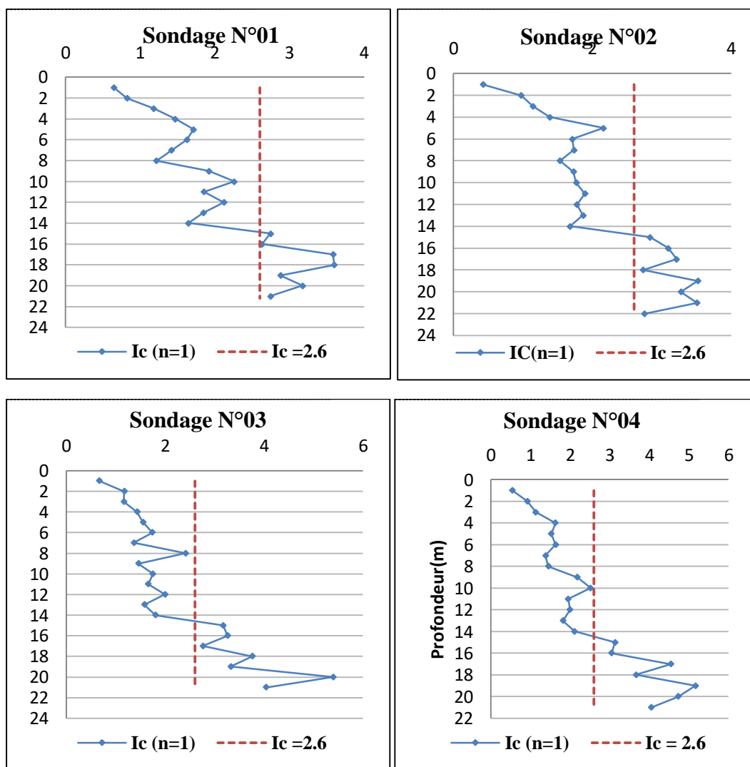
Figure 32: Profile de I_c ( n=1 ) des sondages N°01, 02, 03 et 04
