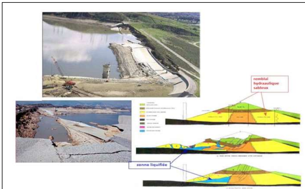
Figure 1.3: Effondrement du parement amont du barrage de San Fernando pendant Le séisme de 1971
