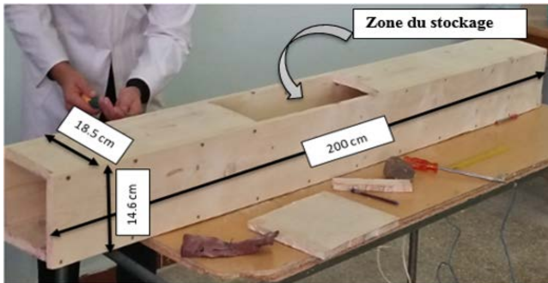
Fig. III.3. Montage du canal de stockeur.
