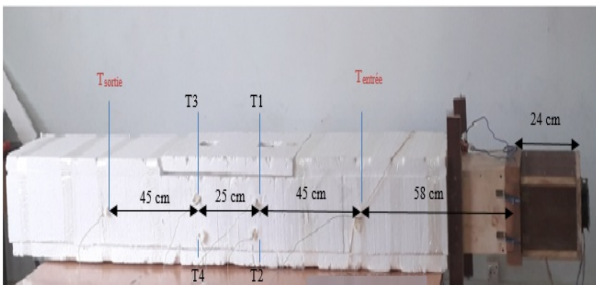
Fig. III.15. Emplacement des thermocouples.
