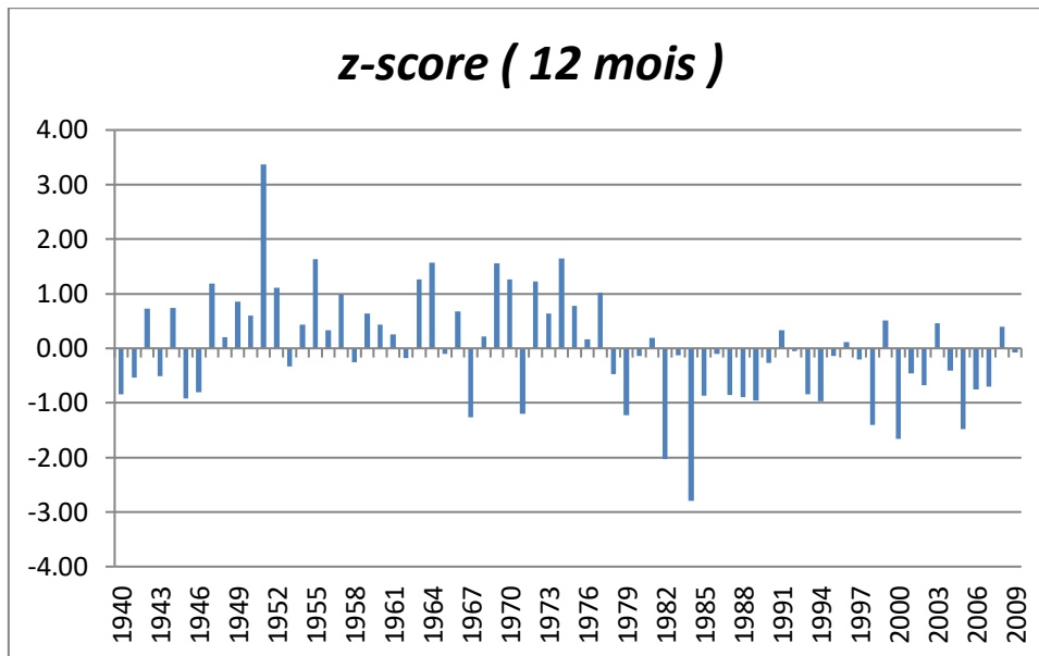
Figure 19 : Evolution du z-score pour des durées annuelles pour la station pluviométrique Tlemcen
