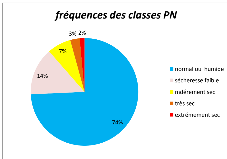
Figure 18 : Fréquence des classes pour PN 12 mois
