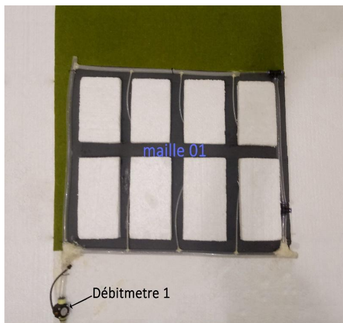
Figure 4.11 : première partie de réseau distribution (maille 01)
