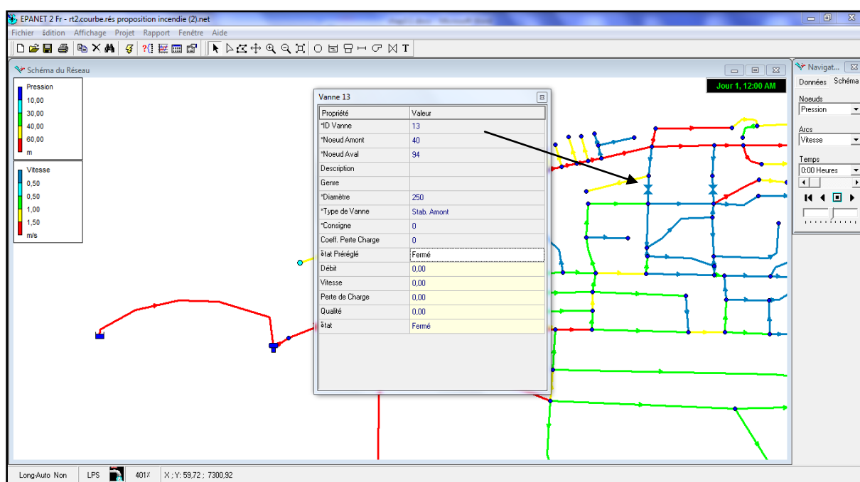
Figure IV.39: Les propriétés d'une vanne.
