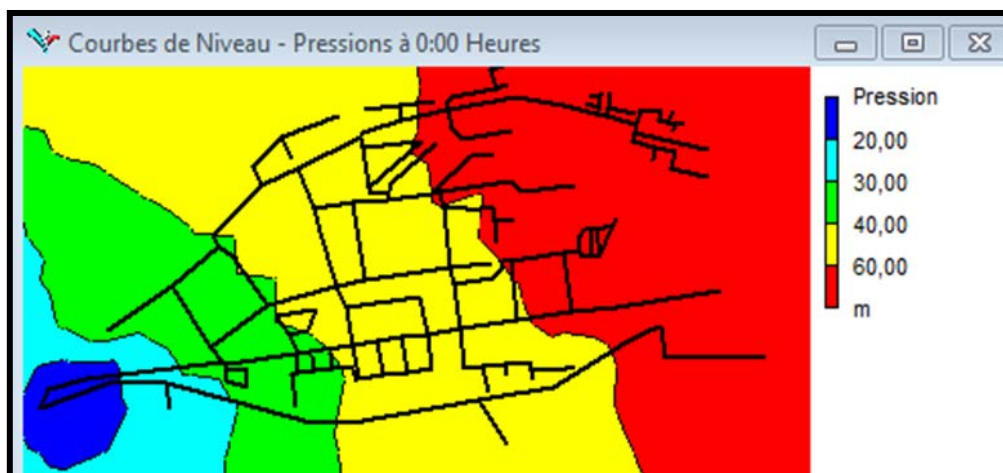
Figures IV.16: L'enveloppe des pressions à l'heure creuses
