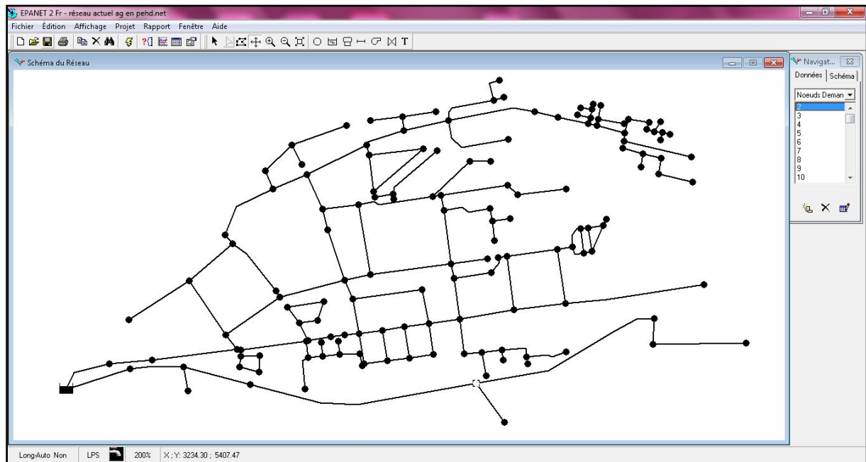
FigureIV.2 : Schéma de réseau actuel de la ville de Remchi sous Epanet
