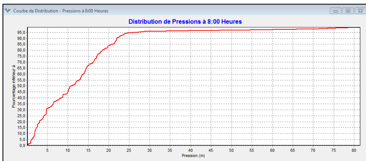
Figure IV.11 : Pourcentage de la distribution de la pression dans les conduites à l'heure de pointe
