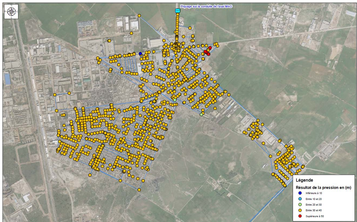
Figure III.12: Résultats de la pression à minuit après sectorisation
