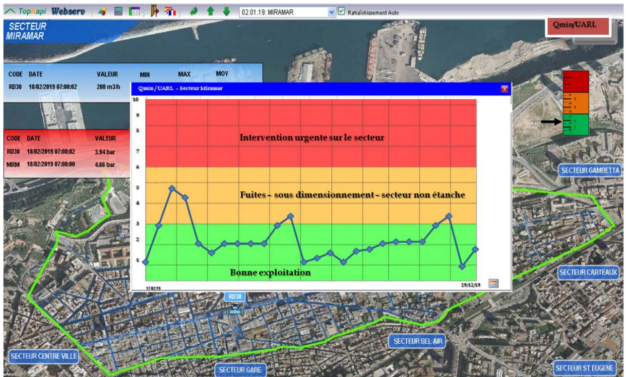
Figure II.4: Affichage journalier du rapport entre le Q nocturne et l'URAL au niveau du service de supervision (SEOR, 2019).
