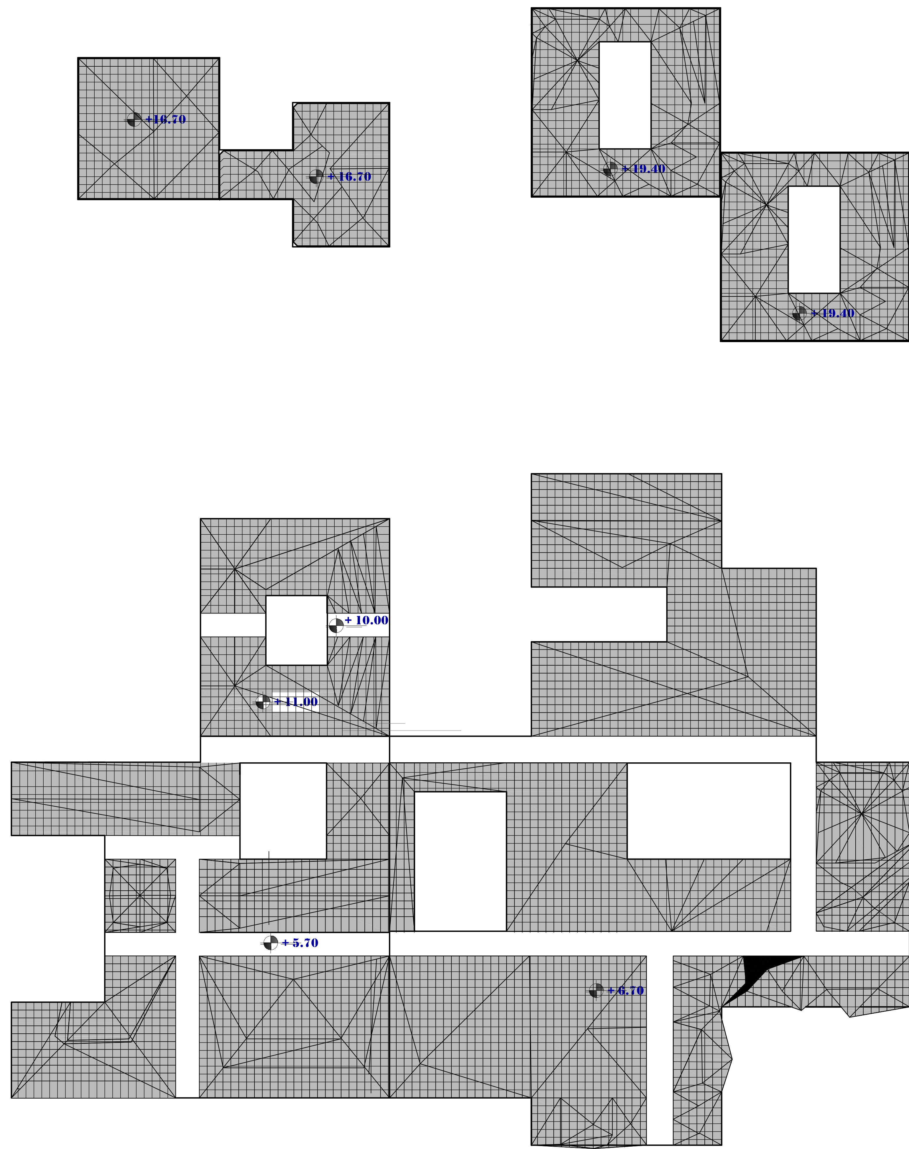
PLAN DE TOITURE ECH 1/200
