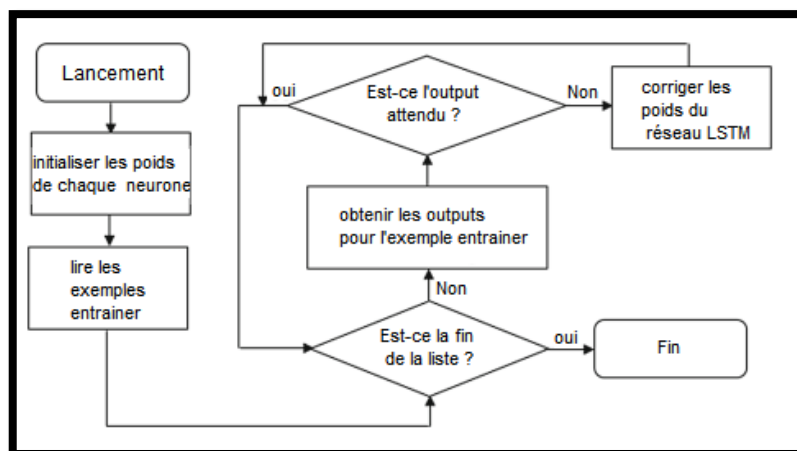
Figure B: Organigramme d'entraînement LSTM.
