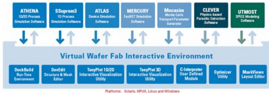
Figure14 : la virtuelle wafer fabrication.
