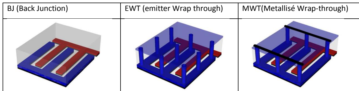
Figure 46: Les cellules a contacte arrière.
