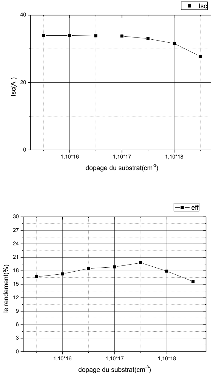
Figure 50 : l'évolution des paramètres principaux de la cellule ewt sous éclairnement en fonction du dopage du substrat
