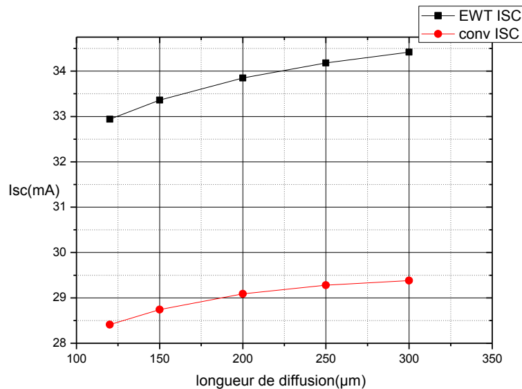
La figure 52 : représenté les résultats de simulation de l'ISC
