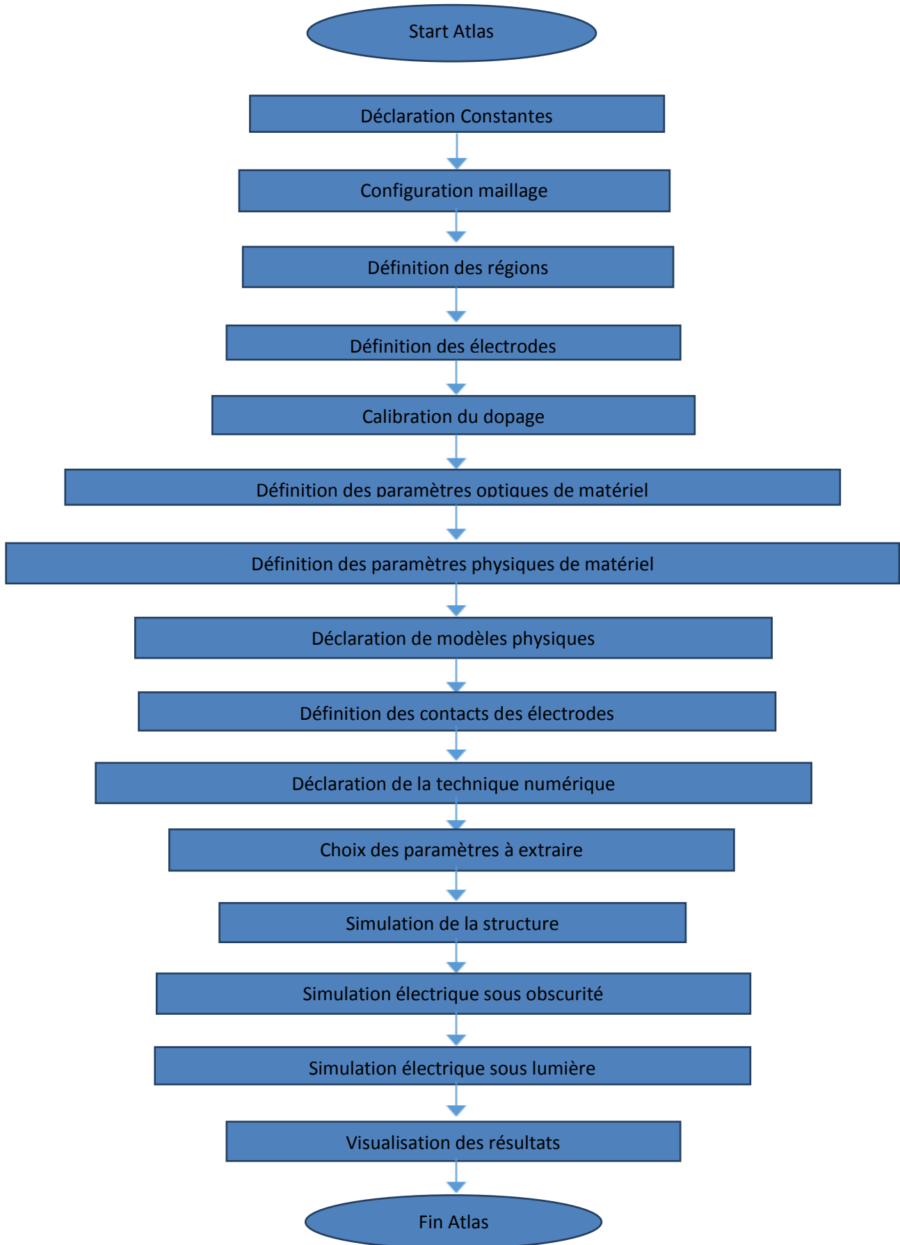
Figure40: Organigramme du programme de simulation
