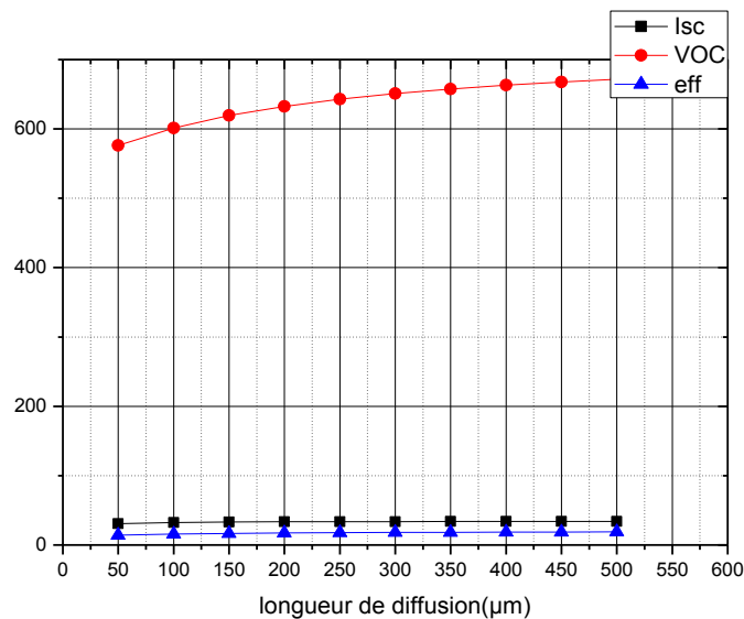
Figure 51 : l'influence de la longueur de diffusion sur le rendement.
