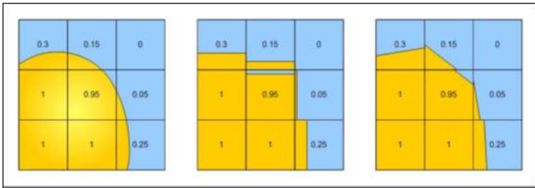
Fig.3.3 Différentes formes de l'interface pour le calcul vof ; (à gauche) Interface réelle et fonction couleur associée ; (au milieu) Classe de méthodes SLIC pour reconstruire l'interface ; (à droite) Classe de méthodes PLIC pour reconstruire l'interface.
