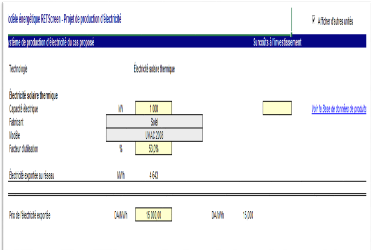
Figure (V.12) : Feuille de calcul modèle énergétique pour les concentrateurs solaires cylindro-paraboliques.
