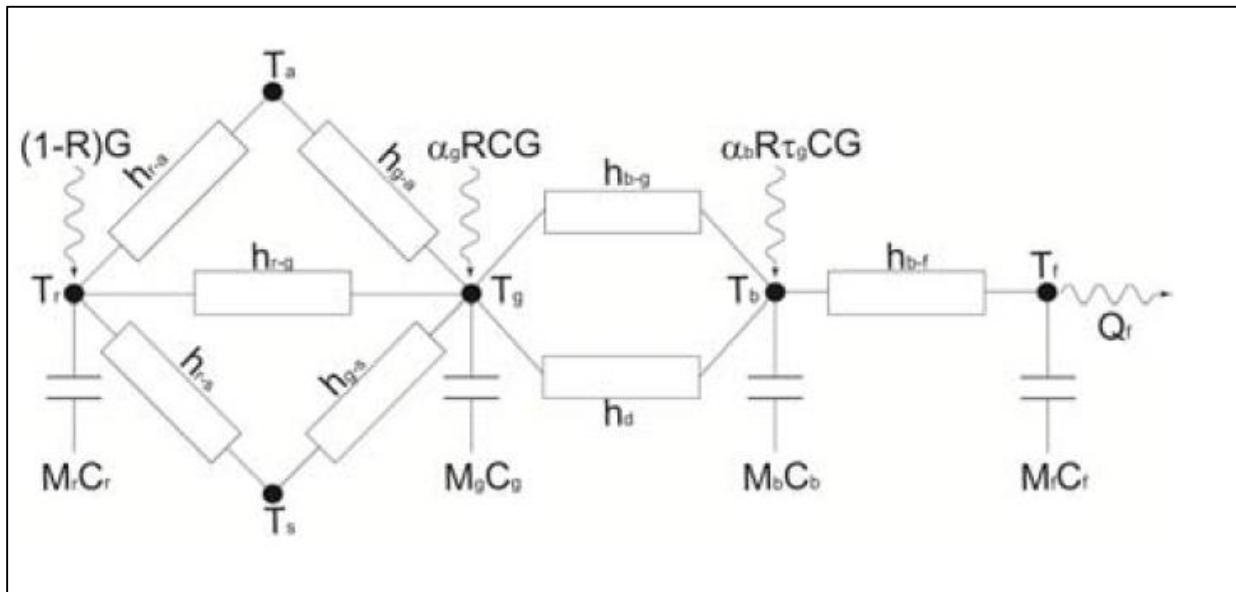
Figure (III.3) : Analogie électrique du problème
