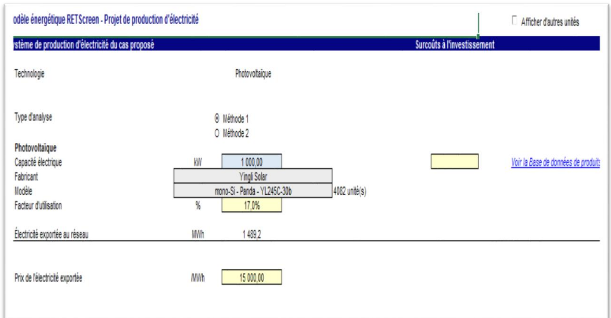
Figure (V.8) : Feuille de calcul modèle énergétique pour le photovoltaïque
