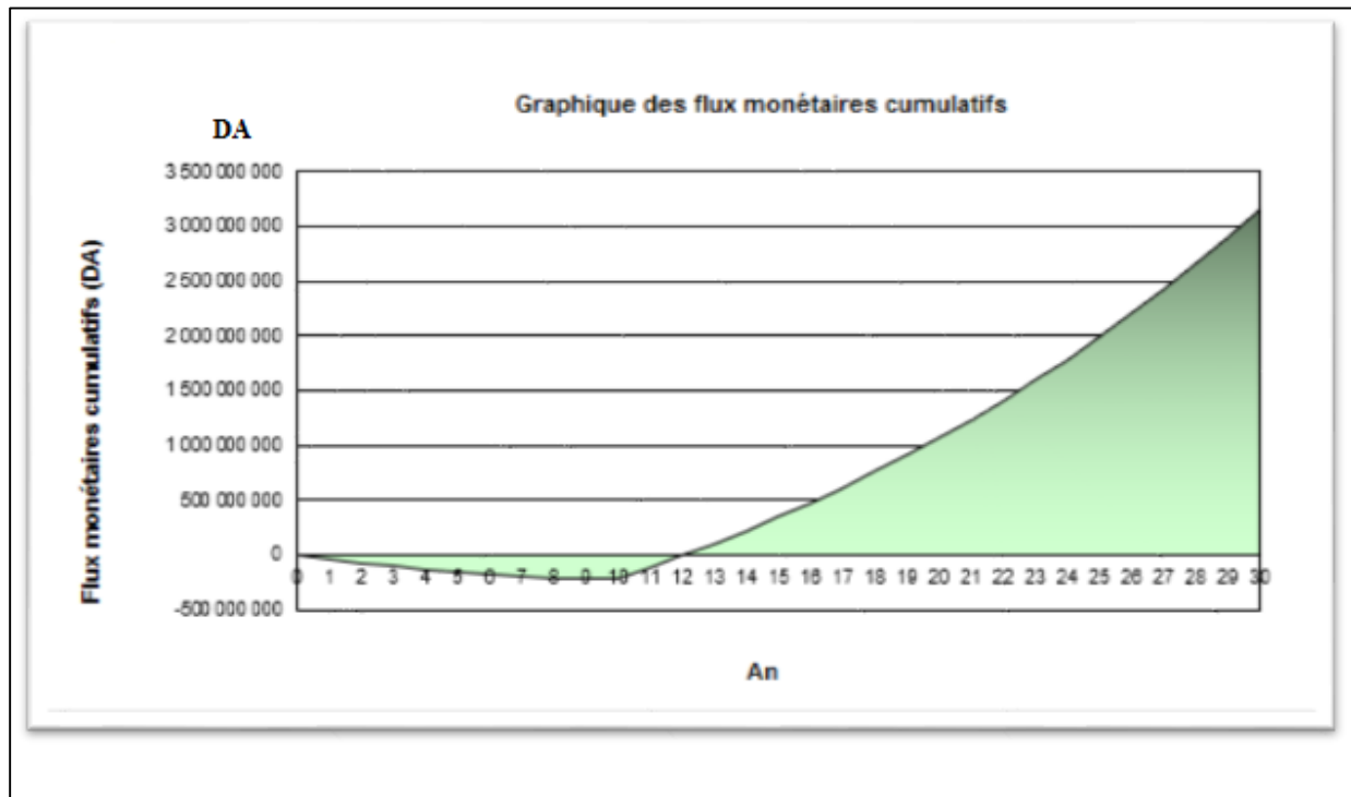
Figure (V.14) : Graphique des flux monétaires cumulatifs pour les concentrateurs solaires cylindro-paraboliques
