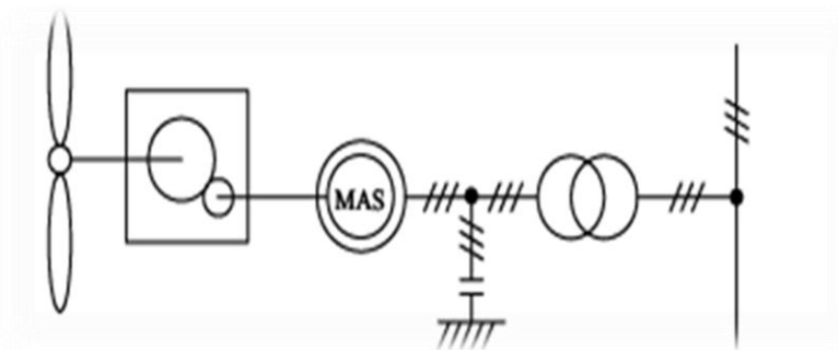
Fig. I.12. Système éolien basé sur la machine asynchrone à cage (vitesse de rotation fixe) [3]
