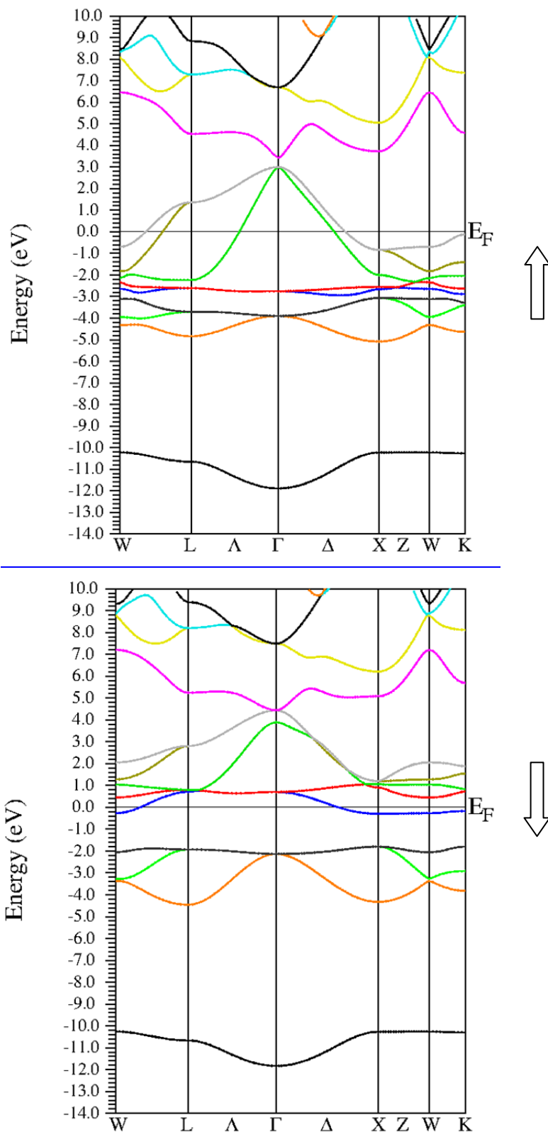
Figure IV.4 : Structures de bandes électroniques (majorité spin et minorité spin) calculées avec la méthode FP-LAPW avec approximation TB-mBJ. L'origine des énergies est prise au sommet de la bande de valence
