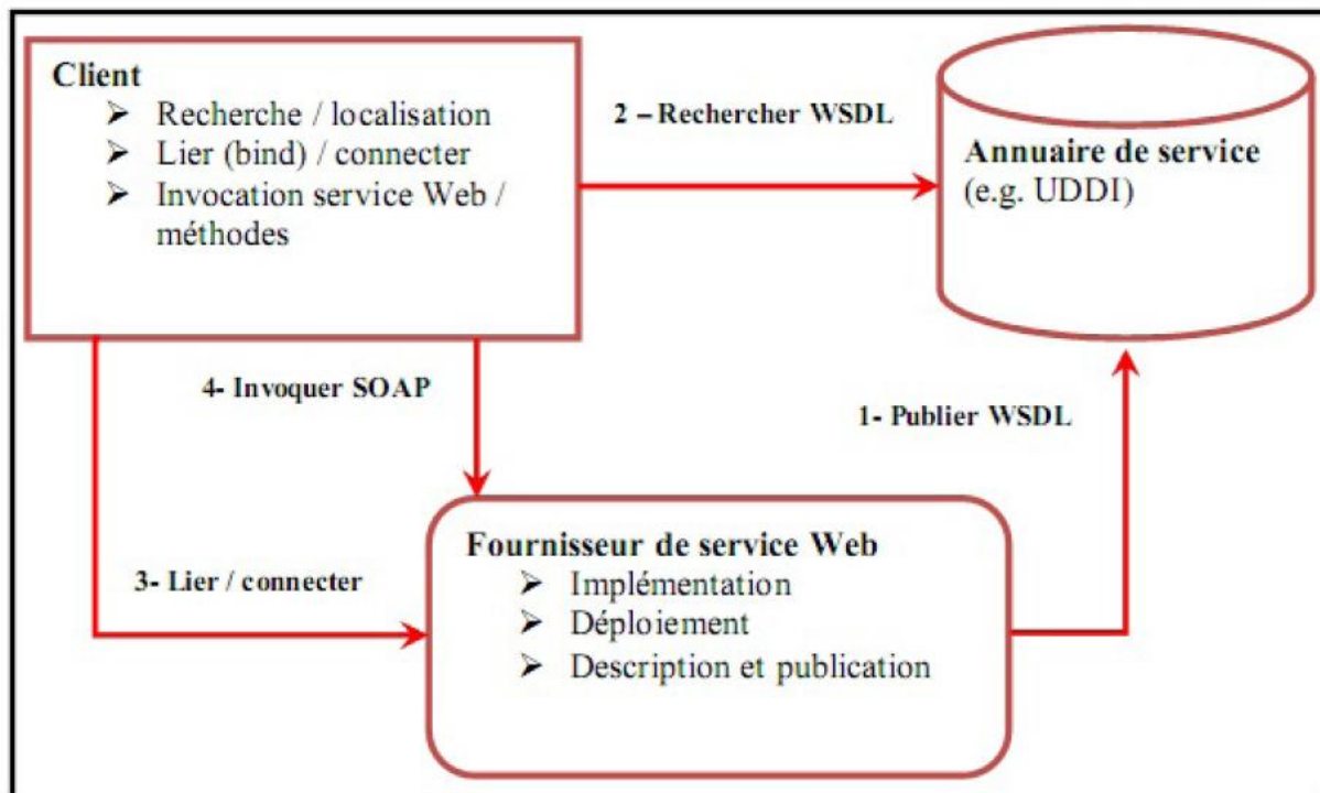
Figure I.1 : Architecture de référence des services Web.
