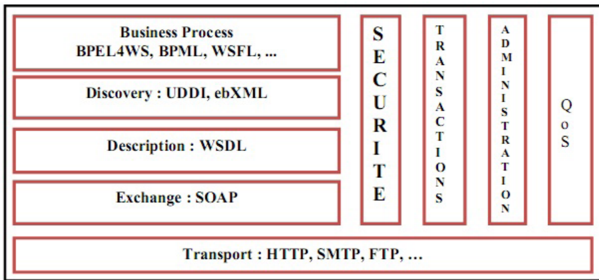
Figure I.2 : Architecture en Pile des services Web.
