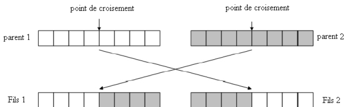
Figure II.6 : l'opération de Croisement
