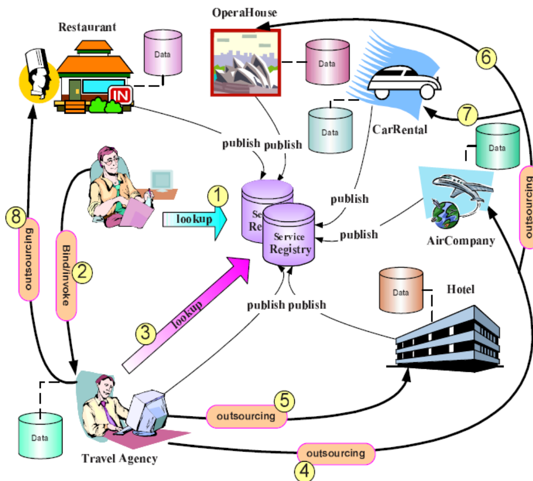
Figure III.1 Un scénario de préparation de voyages
