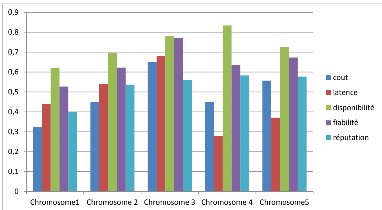
Figure III.8 Histogramme d'optimalité
