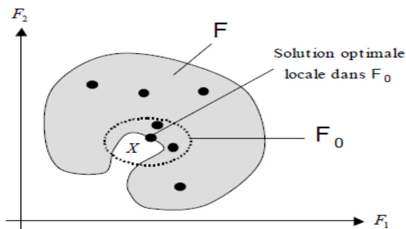
Figure II.3 : Optimalité locale au sens de Pareto
