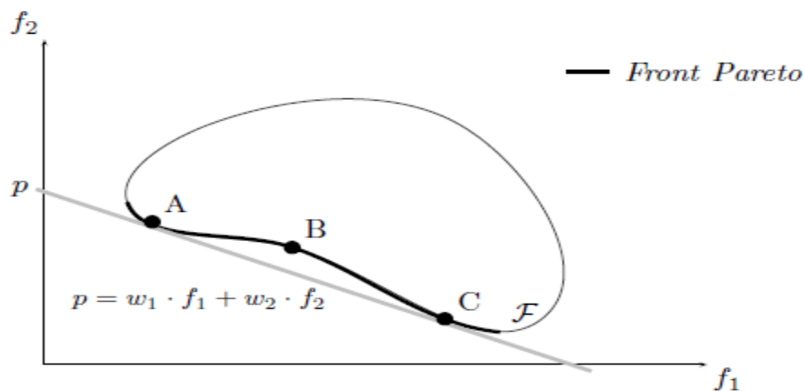
Figure II.4 Interprétation graphique de l'approche par pondération.
