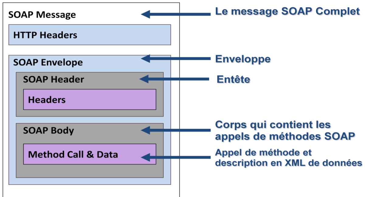
Figure I.4 : les composants d'un message SOAP
