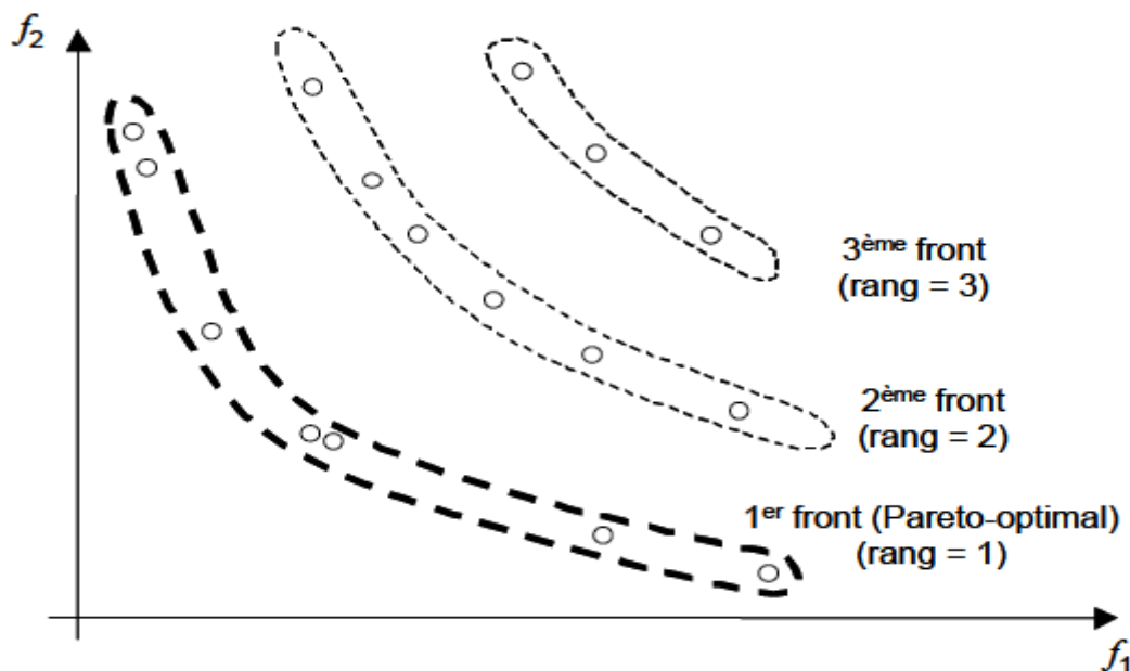
Figure II.8 : Classification des individus selon le rang de Pareto
