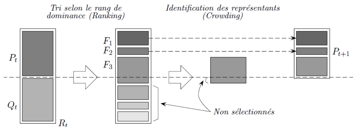
Figure II.10 Fonctionnement de NSGA-II [Deb, 2001].
