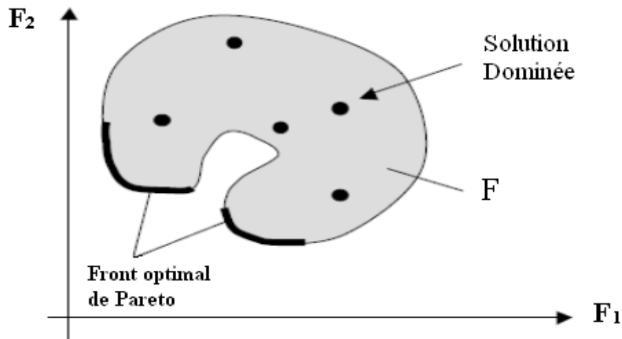
Figure II.2 : Optimalité globale au sens de Pareto
