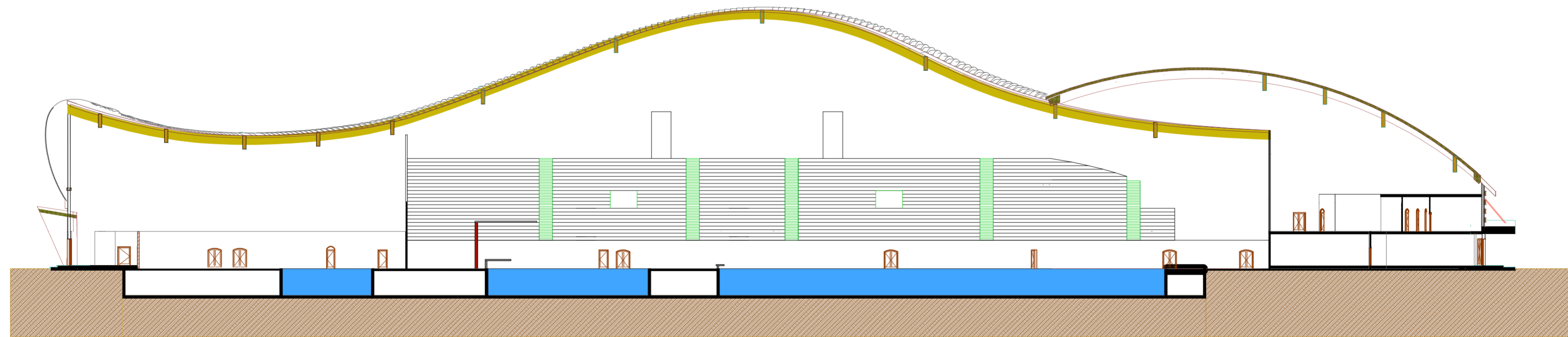
Coupe A-A
