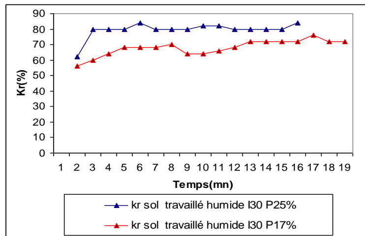
Figure 33 : effet de la pente sur la pluie d'imbibition, le ruissellement du sol travaillé humide (intensité : 30 mm/h ; pente : 17 et 25%)
