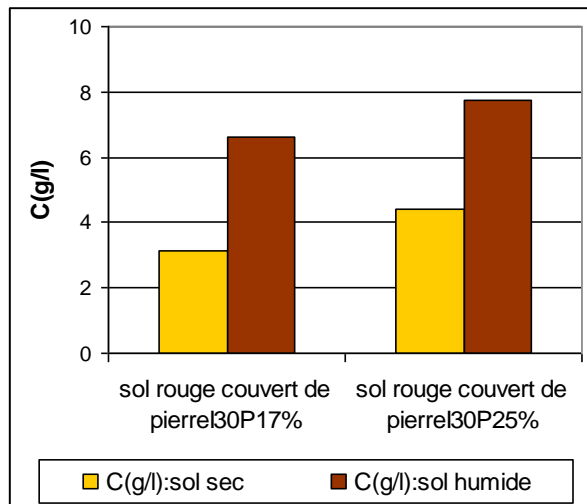
Figure 28 : effet de la pente sur la concentration
