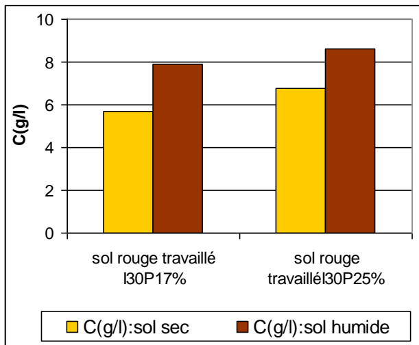
Figure 28 : effet de la pente sur la concentration
