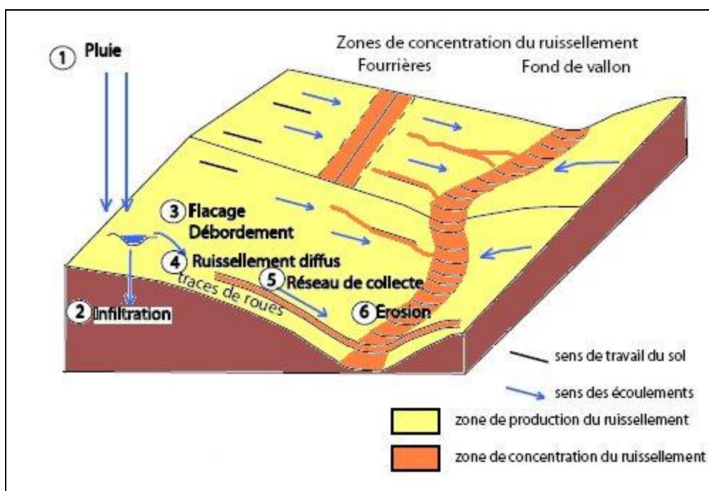
Figure 1 : schéma et processus simplifié de l'érosion (Bussière, 1996)
