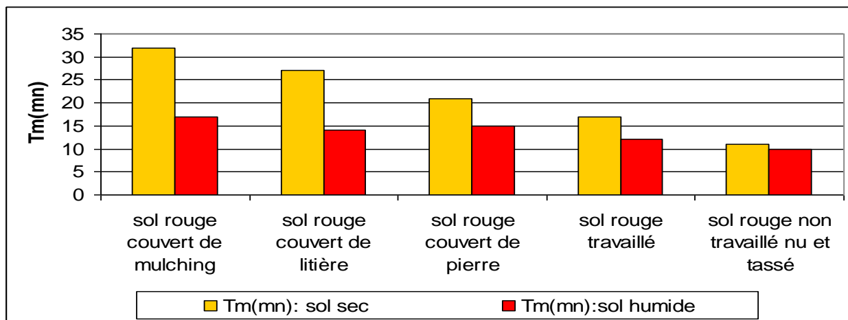
Figure 22 : effet de l'état de sol sur la phase de transition (Intensité : 50mm/h ; pente : 25%)
