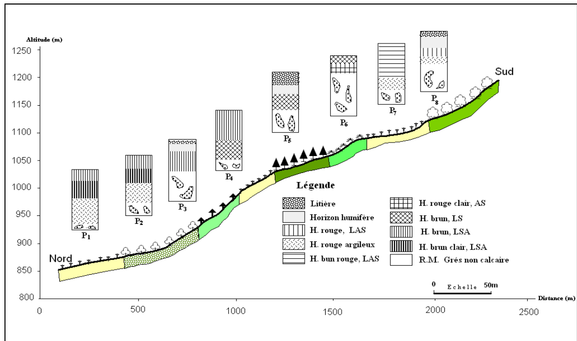
Figure 7 : toposéquence sur substrat gréseux dans la zone de Zariffet ; La variation de la dynamique du sol dû aux processus érosifs est liée à la variation d'occupation du sol (Morsli et al., 2011)
