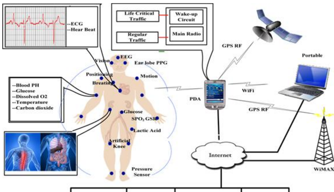
Figure I.4 Réseau WBAN [17].
