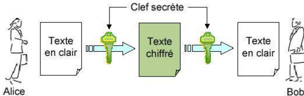
Figure II.1 cryptage/décryptage symétrique [20].
