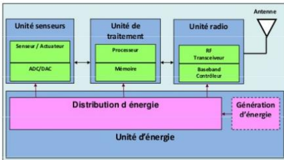
Figure I.2- Architecture d'un nœud de capteur [10].
