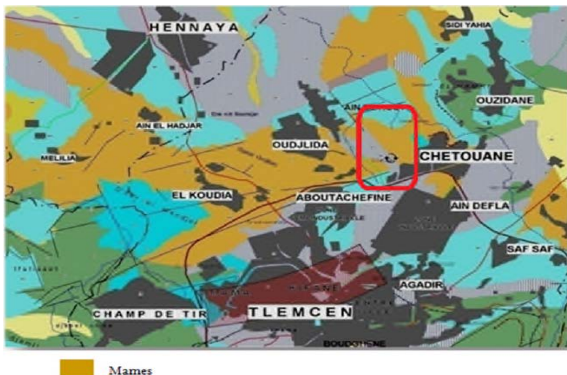
Figure III.3 : Carte géologique Faisant ressortir la constitution du sol de Chetouane (in [19]).
