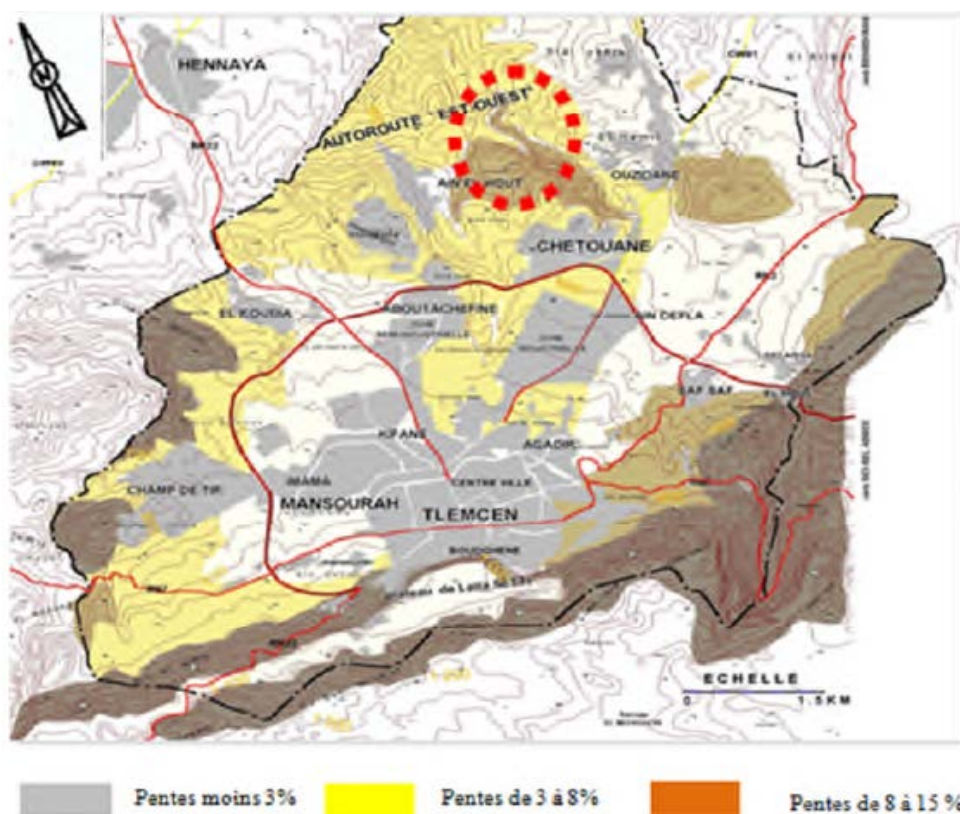
Figure III.2: Pente au niveau de la zone d'étude (in [19]).
