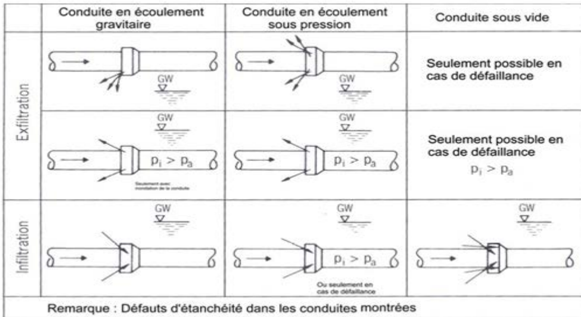
Figure II.2 : Possibilités d'exfiltration et d'infiltration dans les réseaux d'égouts [13].
