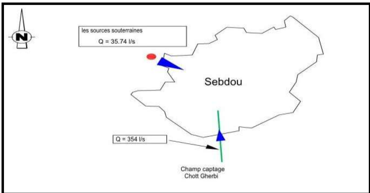
Figure IV.13: Schéma représentant la production totale des eaux alimentant Sebdo.
