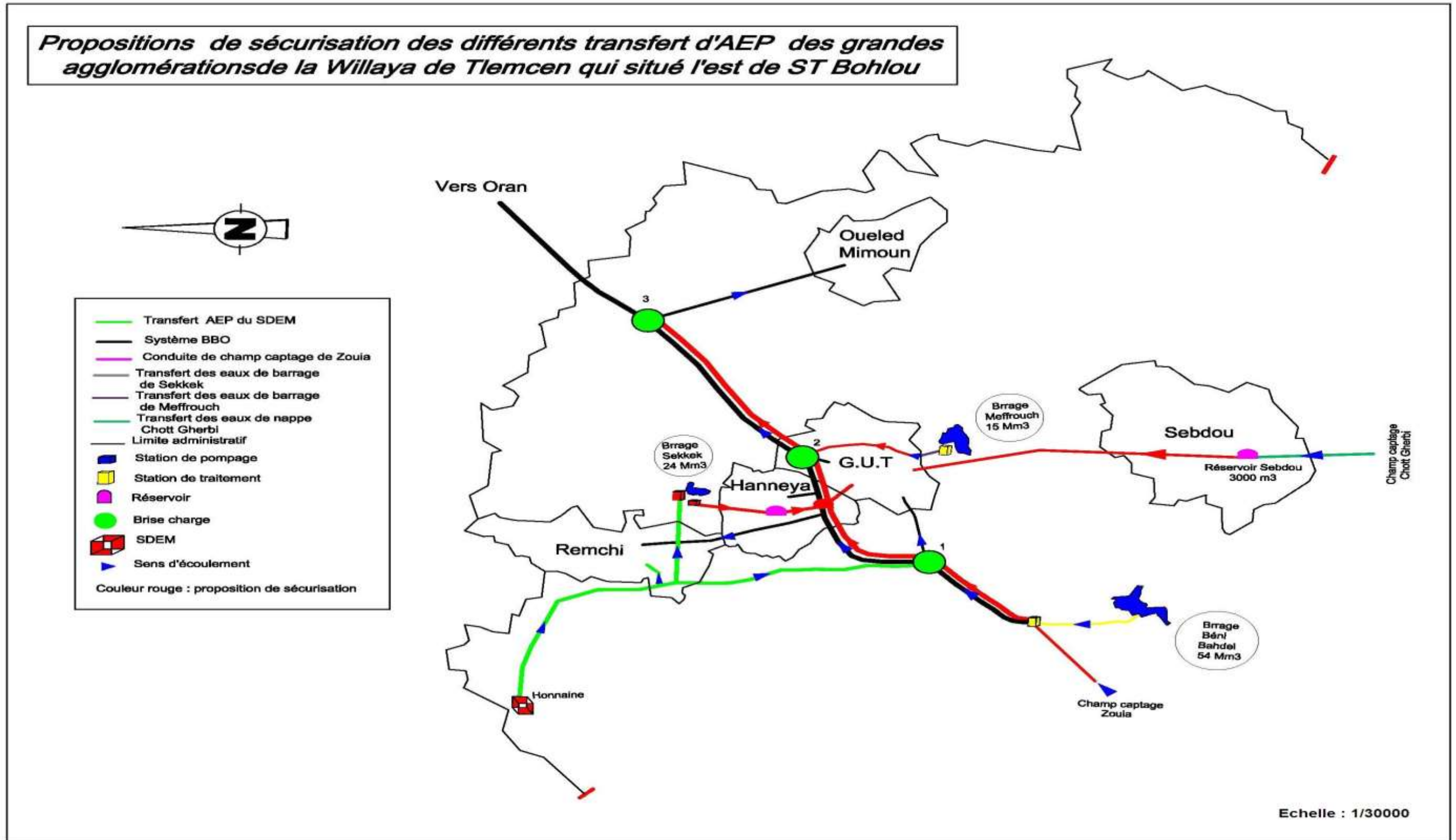
Figure IV.17: Propositions du sécurisation des agglomération situées a l'est de ST Bohlou
