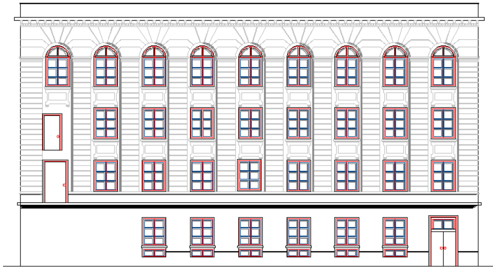
Plan du facade interne
