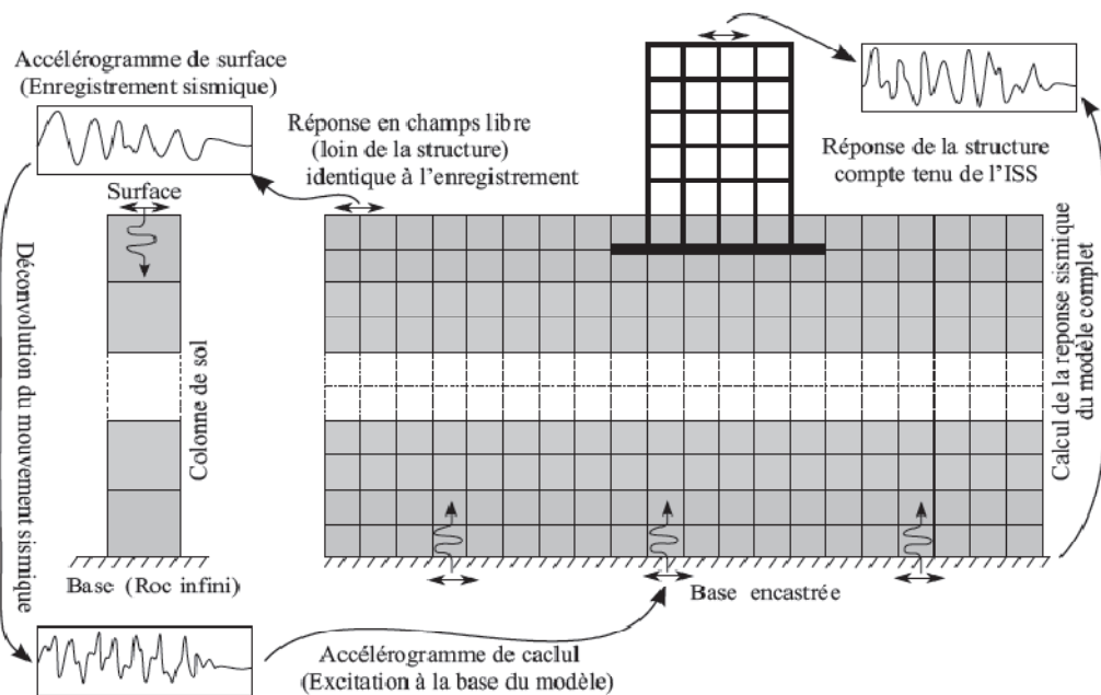
Figure 1. 7: Modélisation de l'ISS par la méthode globale [16].
