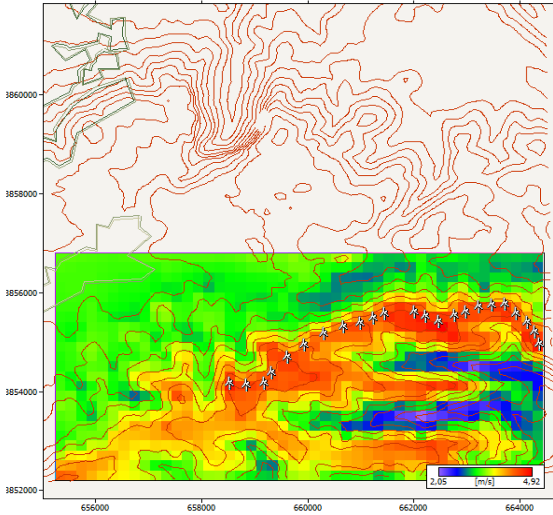
Figure 5-23 . Disposition des éoliennes dans un parc d'une capacité de 18,4 MW
