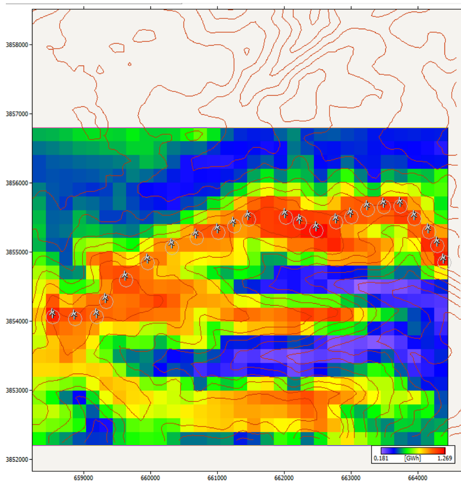
Figure 5-25. Vue sur la disposition des éoliennes sur la carte de l'évolution de la production énergétique annuelle de l'éolienne Nordex N50
