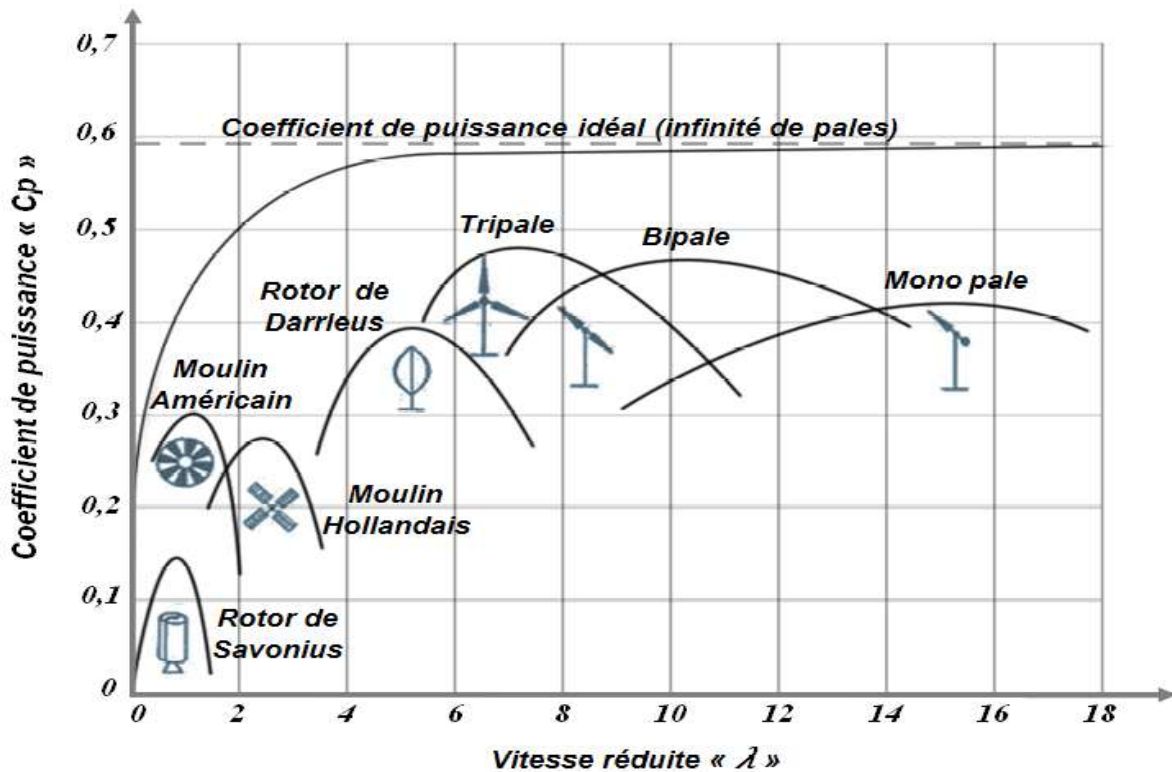
Figure 2-4. Courbes caractéristiques des aérogénérateurs [10]
