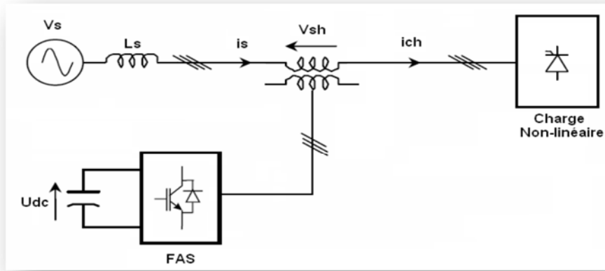
Figure I.3 Filtre actif série [3]
