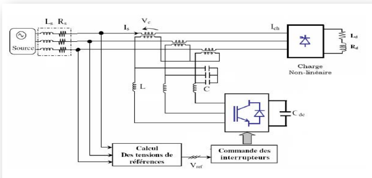
Figure II.2 Schéma de principe d'un filtre actif série [11]
