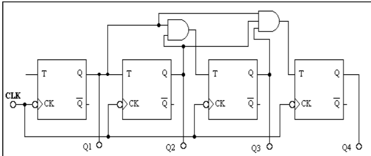
Figure 1.34 : Compteur synchrone 4 bits.
