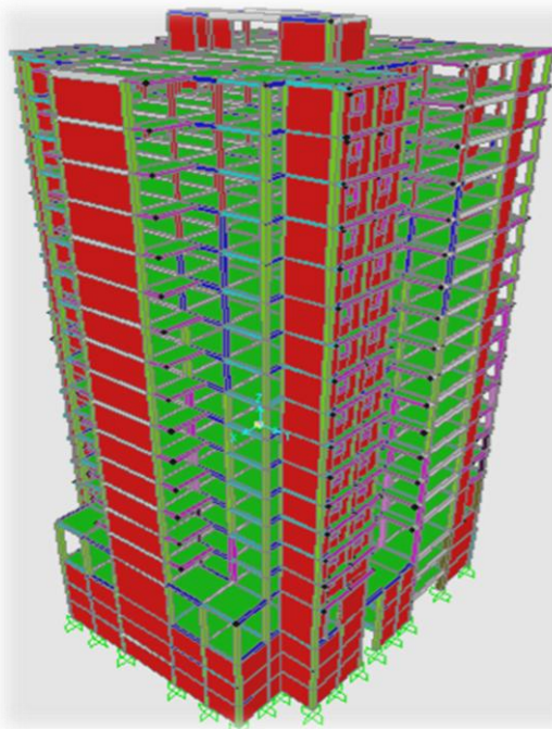
Figure V.1. Modèle 3D de la structure
