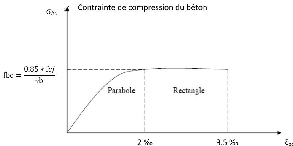
Figure I. 3 : Diagramme contraintes- déformations du béton
