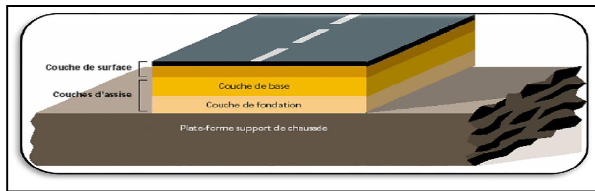
Figure 3.1: Structure type d'une chaussée souple. [17]
