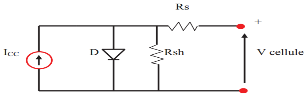
Fig 1: Schéma électrique d'une cellule photovoltaïque
