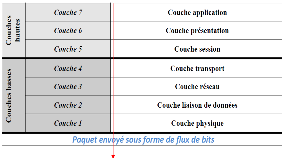
Figure I.1 : Les couches du modèle OSI. [2]
