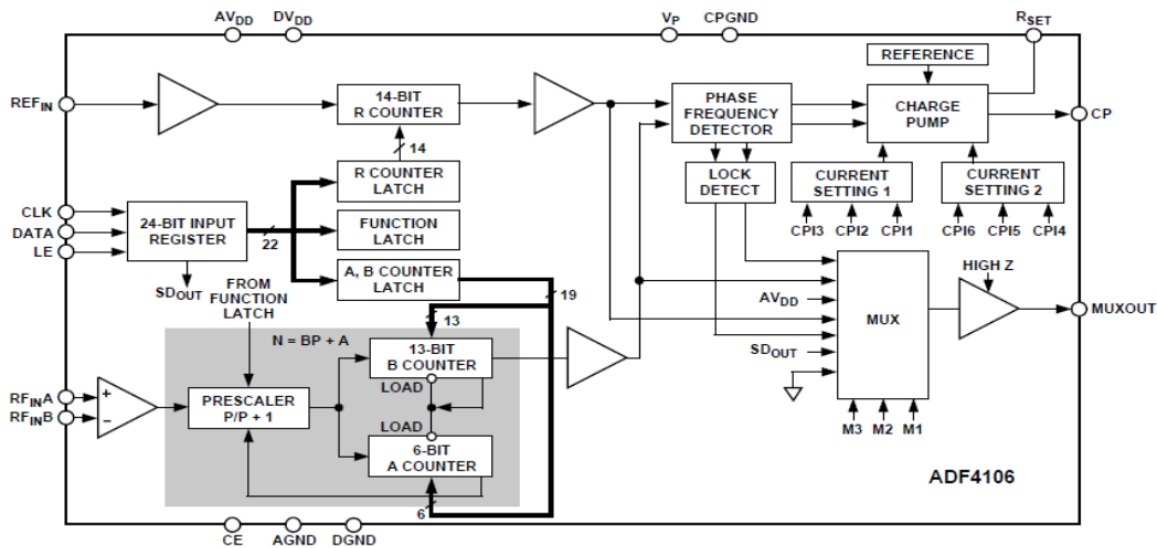
Figure IV.2. Schéma fonctionnel de l'ADF 4106 [45].
