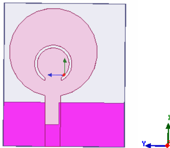
Figure III.19. antenne avec résonateur en anneau fendu circulaire.
