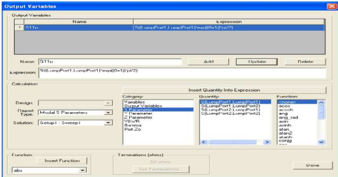
Figure III.5: Définition d'un variable non prédéfinie sur HFSS [3].
