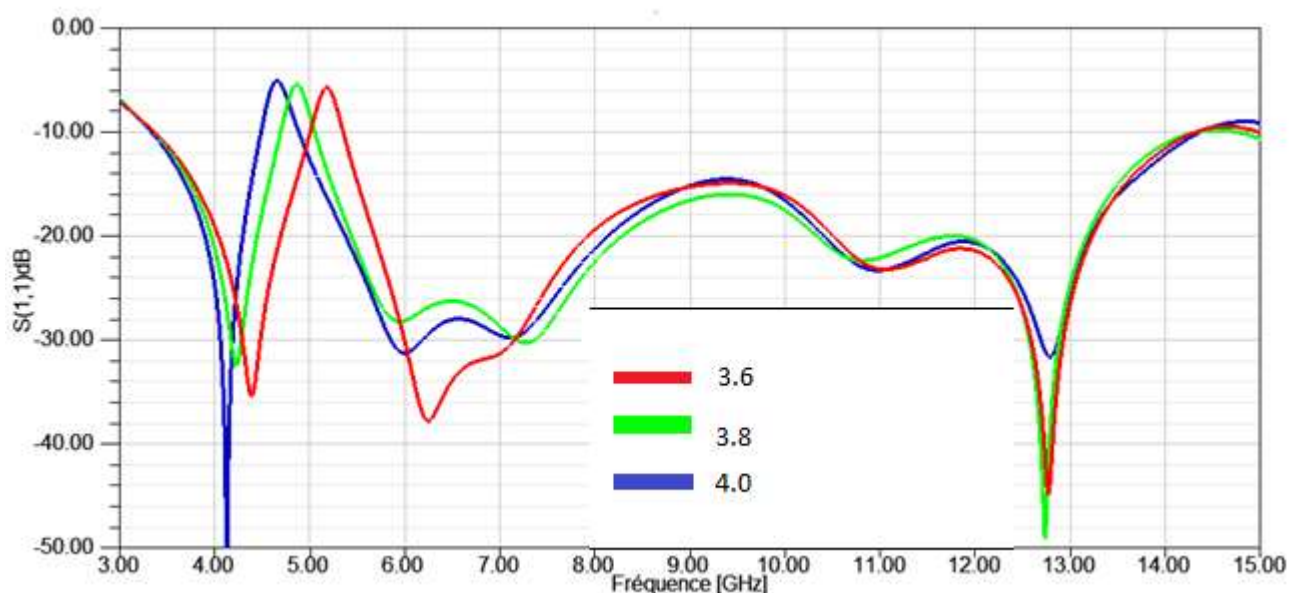
Figure III. 20. Variation du coefficient de réflexion pour les différentes longueurs en fonction de la fréquence pour différentes valeurs de Rraf.
