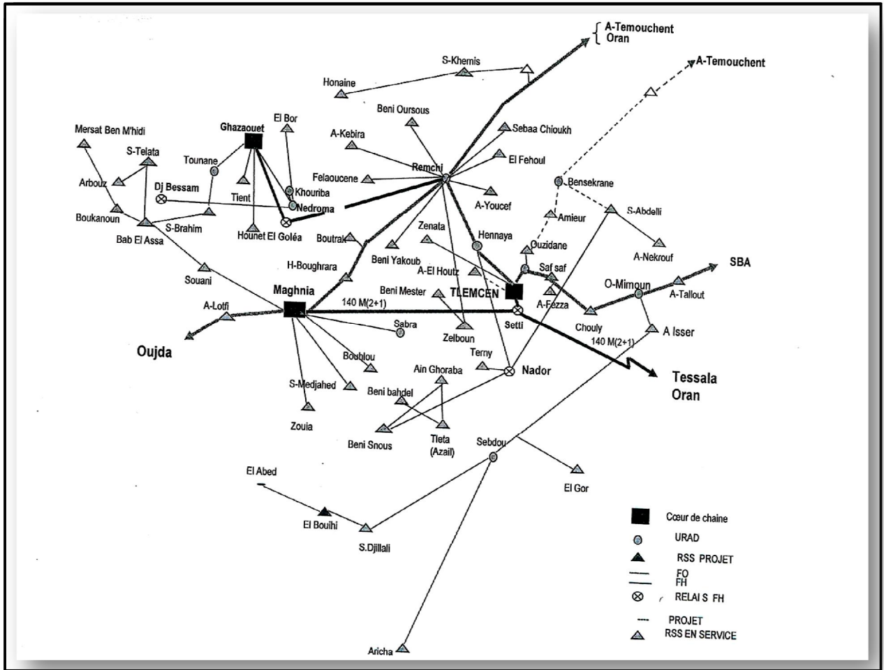
Figure IV.29 : Réseau de transmission de la wilaya de Tlemcen
