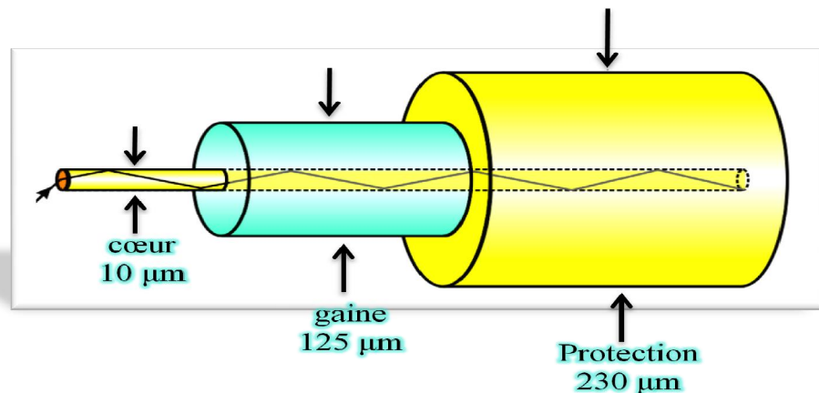
Figure I.5 : Composition d'une fibre
