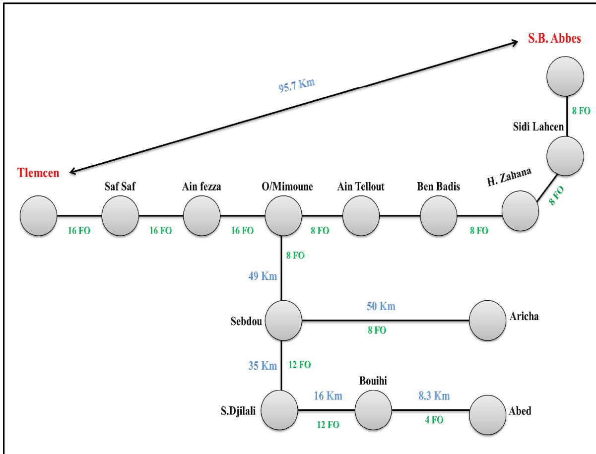
Figure III.1 : FO Tlemcen-S.B.Abbes via O/Mimoune
