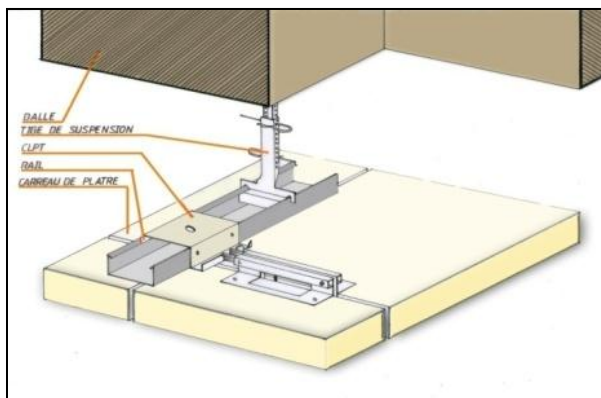
Figure 59: faux plafond
