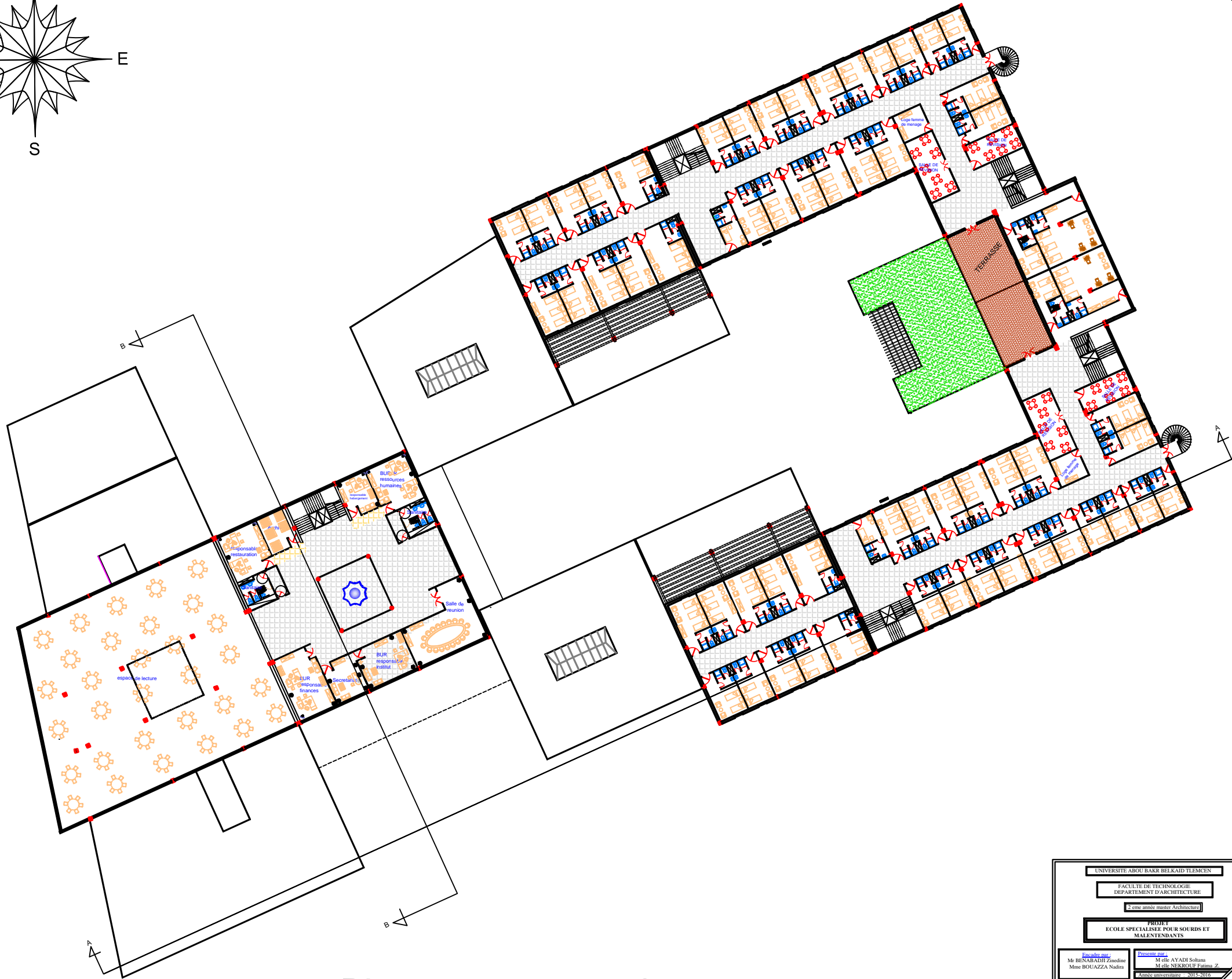
PLAN 3 EME ETAGE ECH : 1/200
