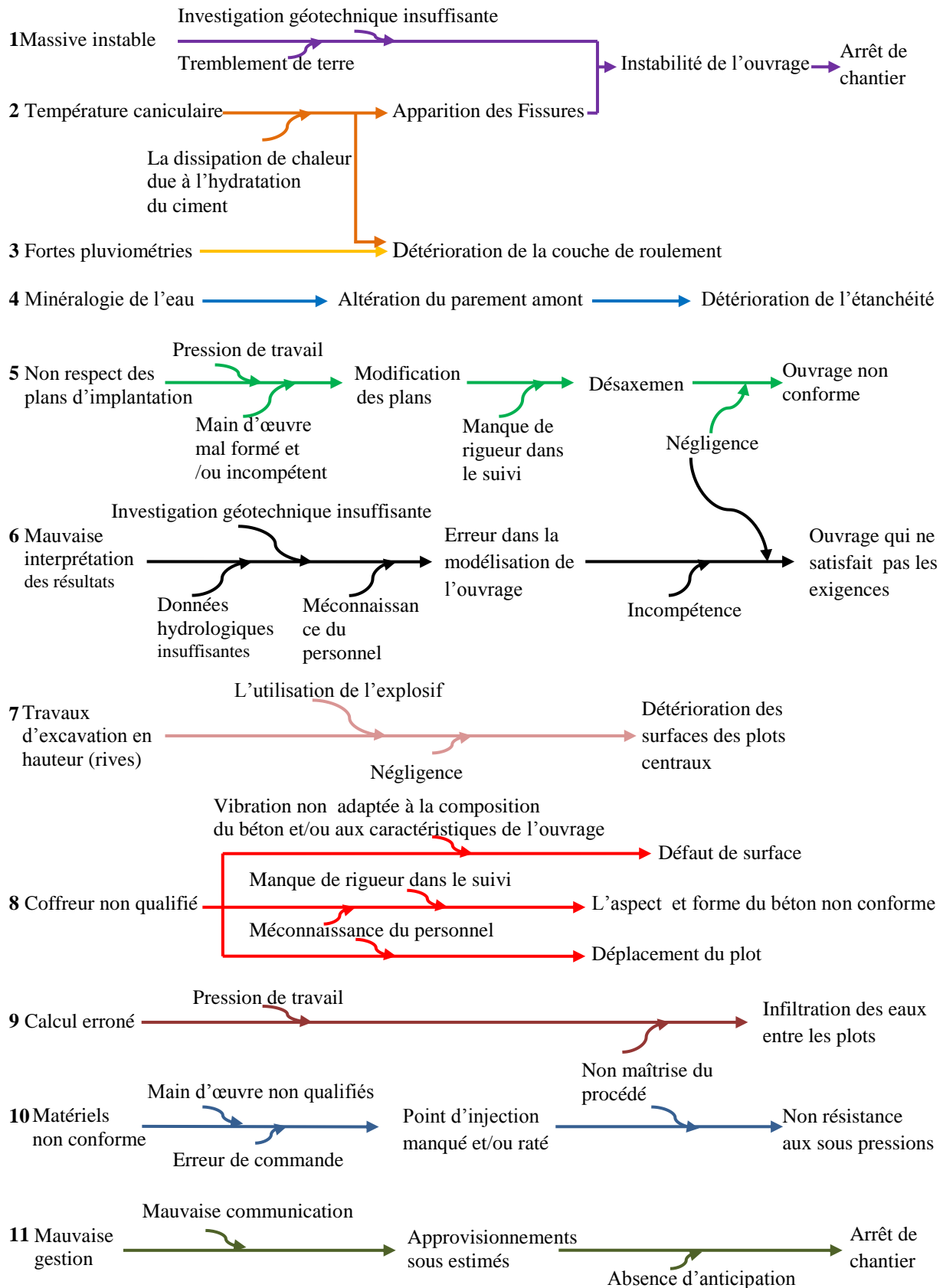
Figure 4.12. Scénario court du SS1 Corps du barrage & Injections
