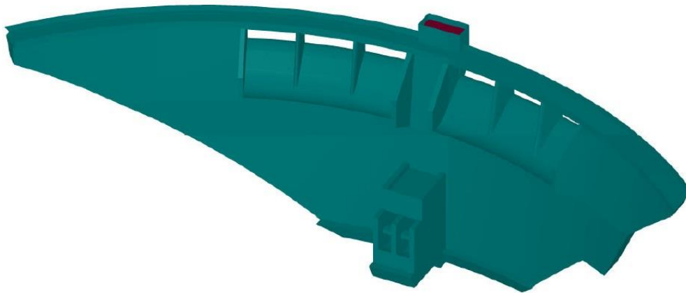
Figure 3.8. Vue 3D du barrage type voûte (vidange représentée); (ISL, 2011)
