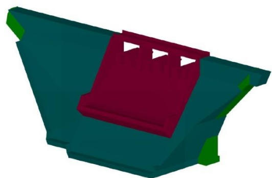
( b ) Barrage en BCR
