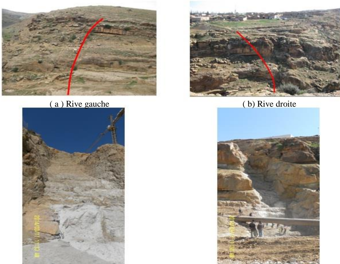
Figure 3.10. Les deux rives du barrage oued Taht avant et après les travaux d'excavation.
