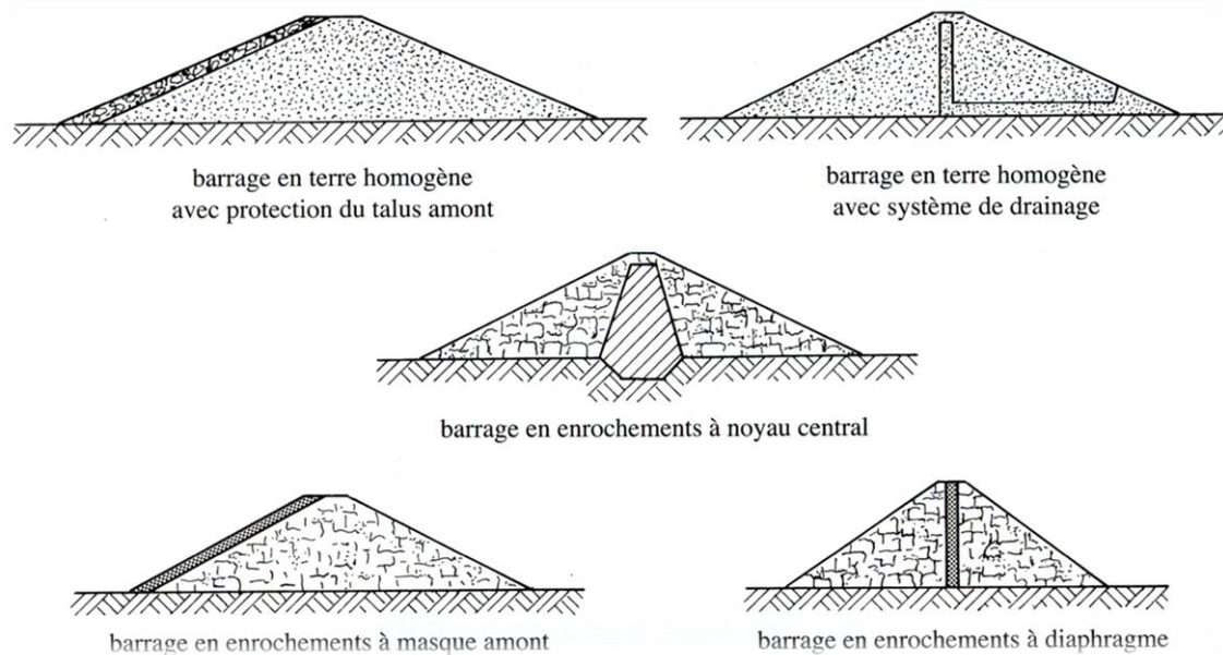
Figure 1.8. Coupes schématiques de différents types de barrages en remblai et disposition des éléments d'étanchéité (SCHLEISS A.J. & POUGATASCH H., 2011).
