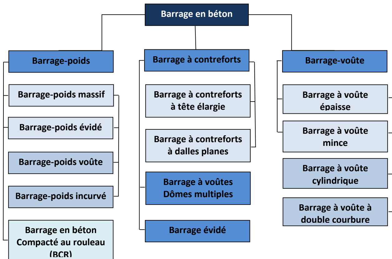
Figure 1.4. Les familles des barrages en béton (SCHLEISS A.J. & POUGATASCH H., 2011).
