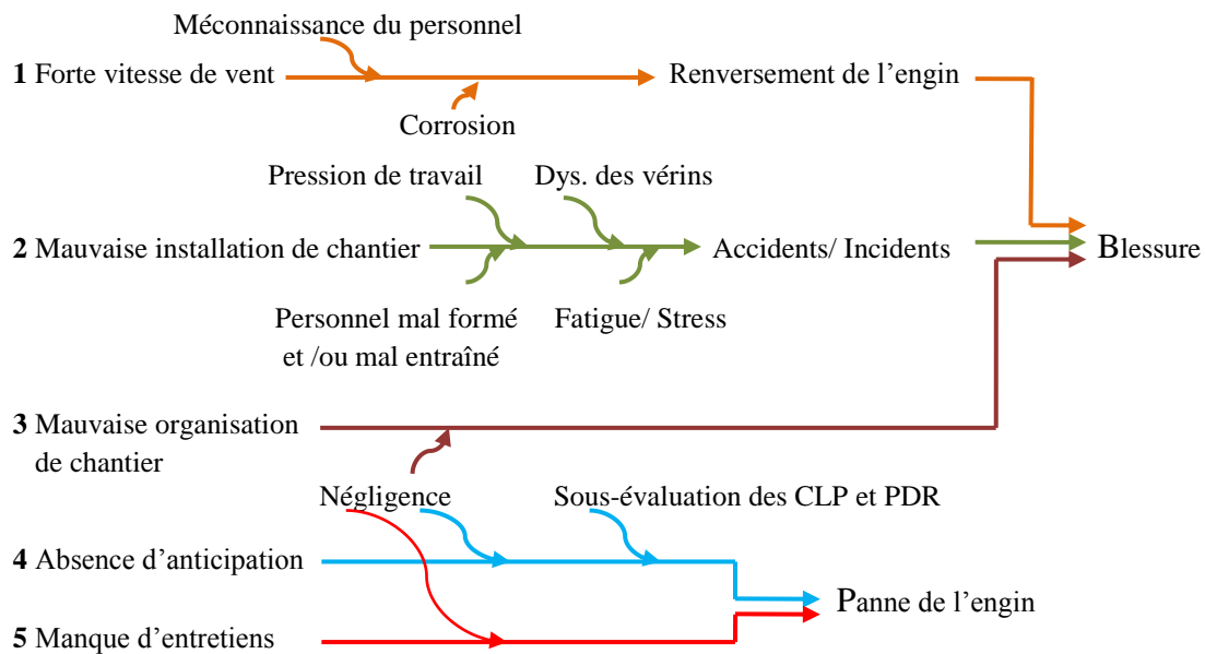
Figure 4.14. Scénario court du SS3 Engins
