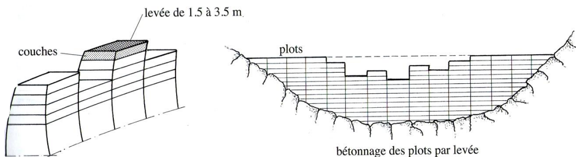
Figure 1.6. Etapes de bétonnage (SCHLEISS A.J. & POUGATASCH H., 2011).
