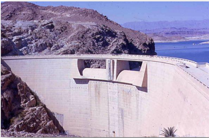
Figure 1.1. Barrage voûte de Foug el Gherzamis en service en 1950, situé à proximité de Biskra (Algérie). Sa hauteur maximale est de 73 m. (Tiré de : www.algerie-verite.com )
