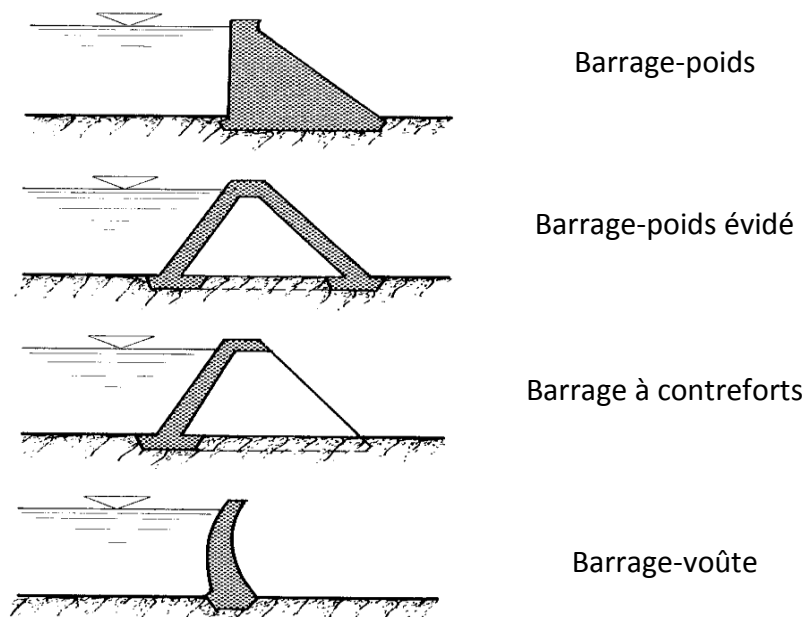
Figure 1.5. Coupes-type des barrages en béton (SCHLEISS A.J. & POUGATASCH H., 2011).
