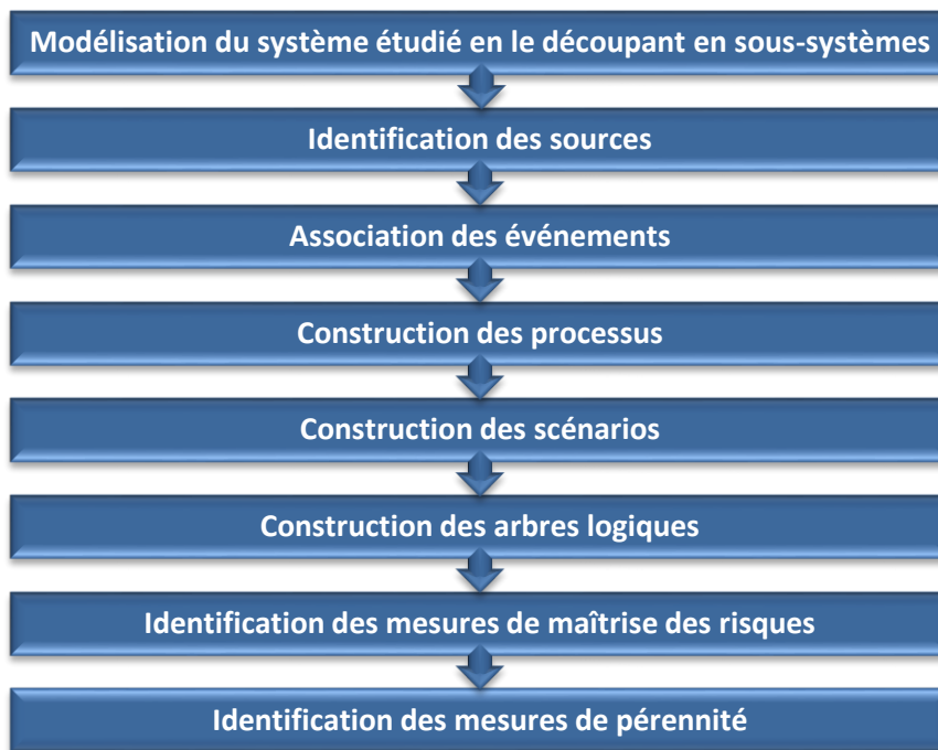
Figure 4.4. Les huit étapes de la mise en œuvre de MADS-MOSAR (GRANDAMS O., 2010).
