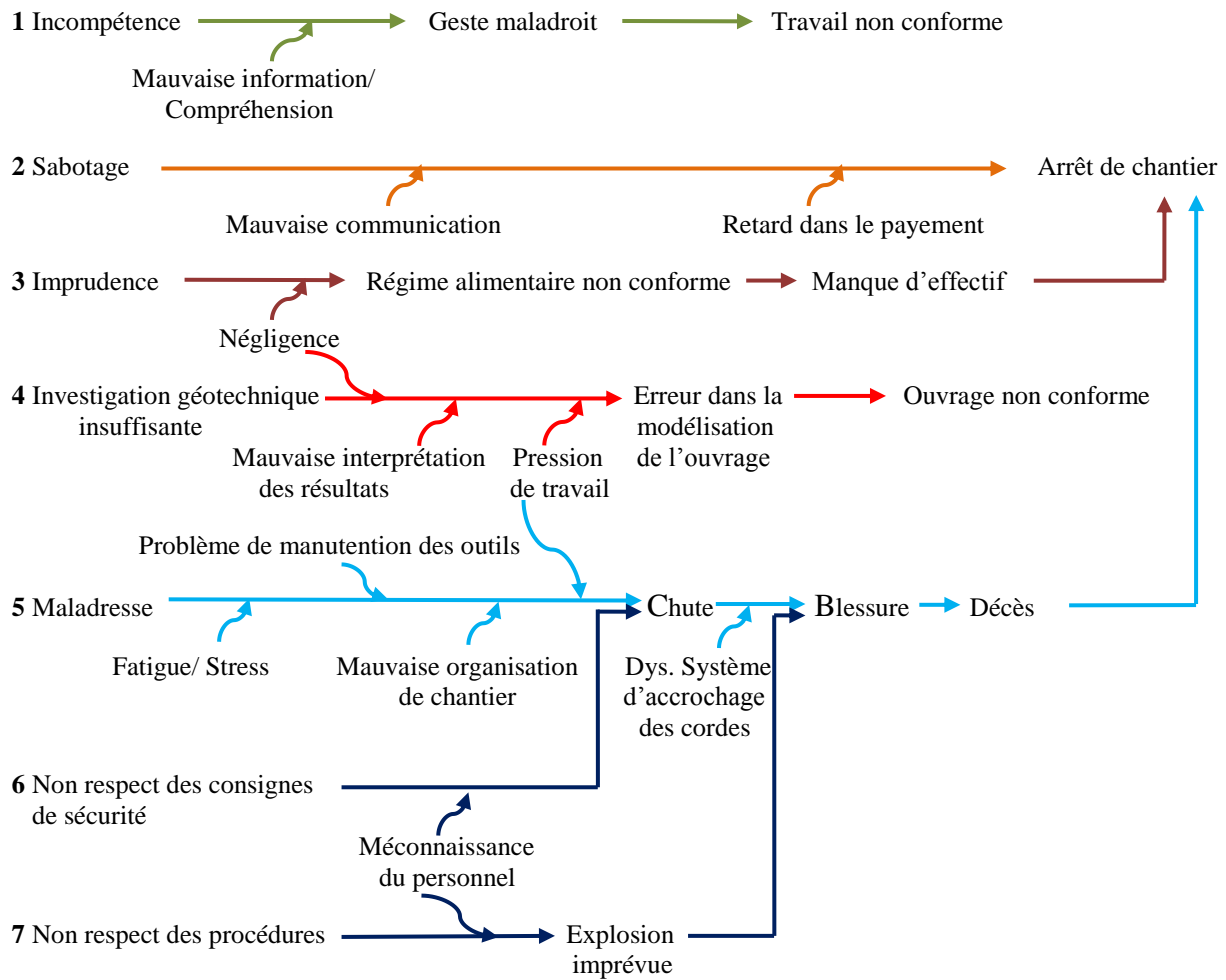
Figure 4.15. Scénario court du SS4 Ressource humaine
