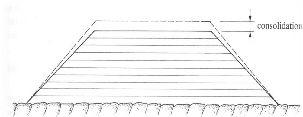
Figure 1.9. Barrage en remblai-mise en place et consolidation (SCHLEISS A.J. & POUGATASCH H., 2011).
