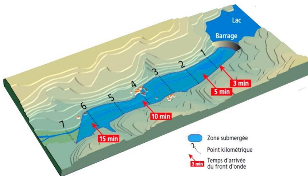
Figure 2.3. L'onde de submersion
