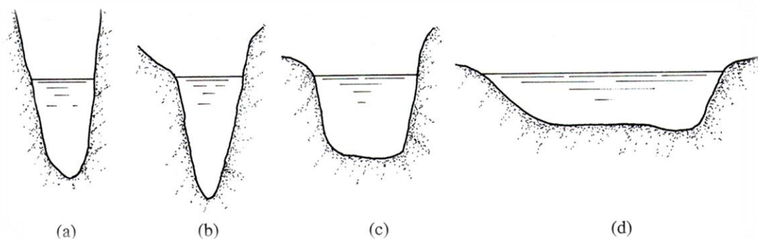
Figure 3.2. Représentation schématique des différentes formes de vallées : (a) Gorge ou canyon ;(b) vallée en V ;(c) vallée en U ;(d) vallée large. (SCHLEISS A.J. & POUGATASCH H., 2011).
