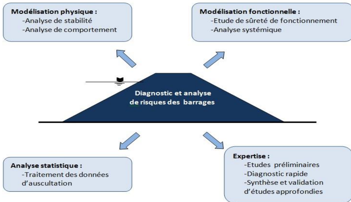
Figure 2.13. Les différentes approches du diagnostic et de l'analyse de risques pratiquées dans le domaine des barrages ((PEYRAS L., 2002)
