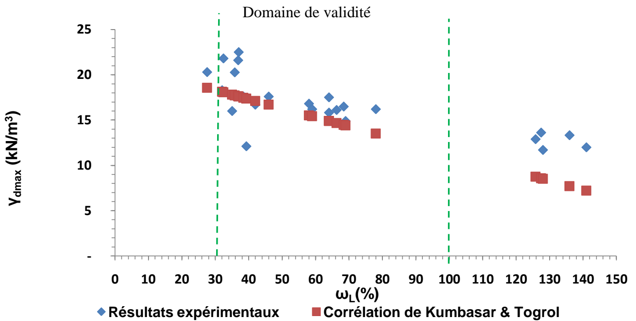
Figure III.19 : Comparaison entre les densités sèche maximales mesurées et estimées par la corrélation de KUMBASAR & TORGOL (1969)
