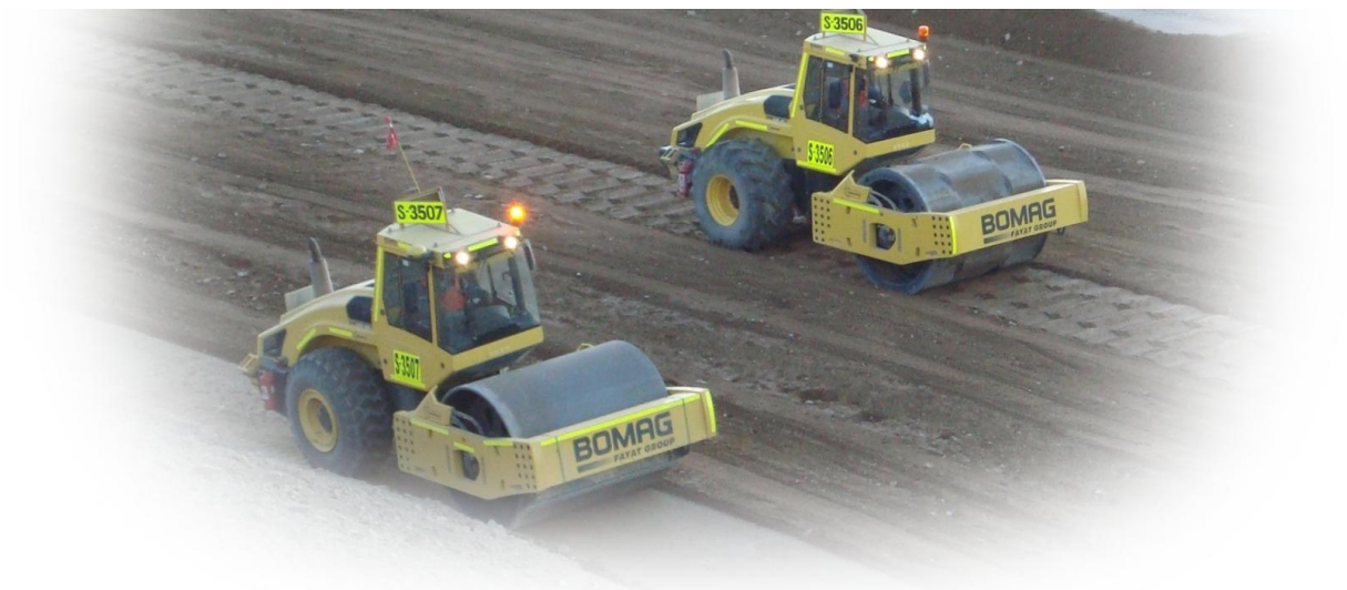
Photo II.2 : L'opération du compactage statique sur un site de construction
