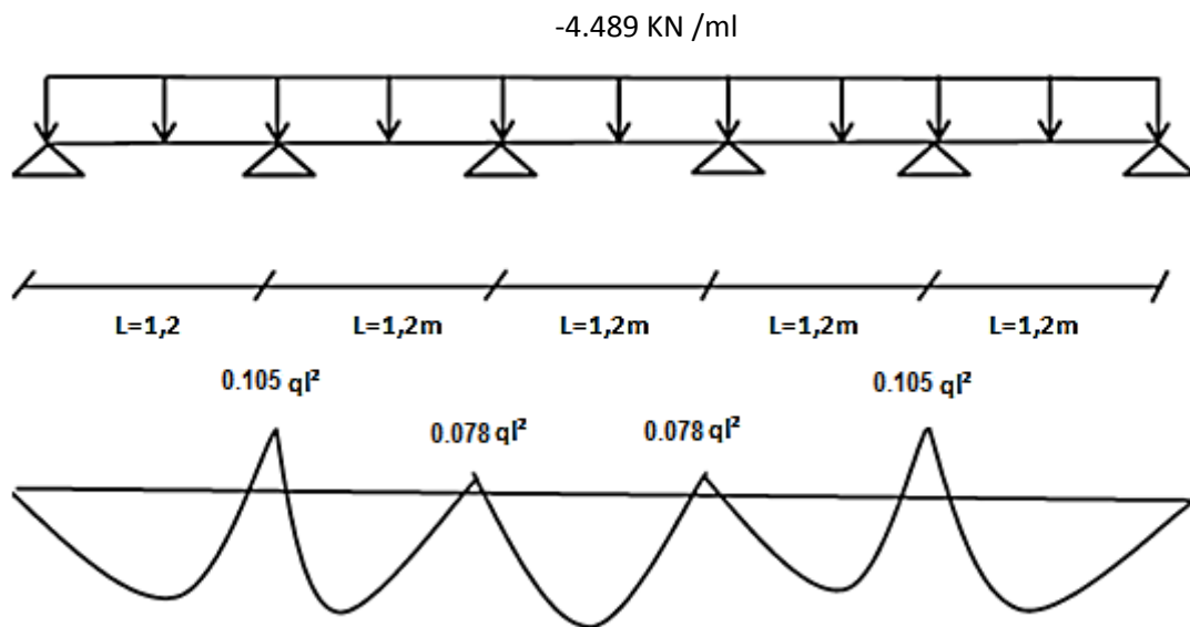
Figure III.4 Diagramme des moments fléchissant au niveau de la couverture
