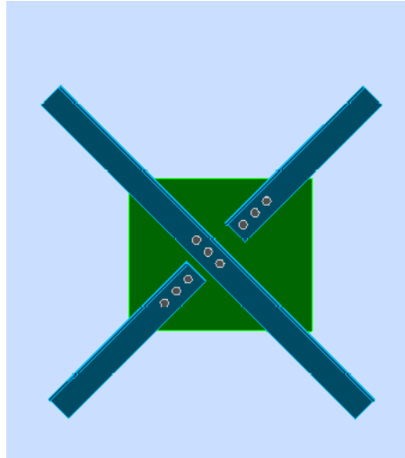
Figure VI.3 vue en 3D de l'assemblage de contreventement
