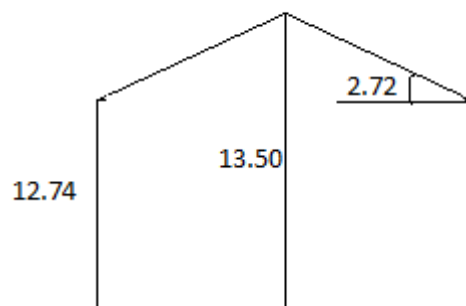
Figure II.4 La pente de la toiture
