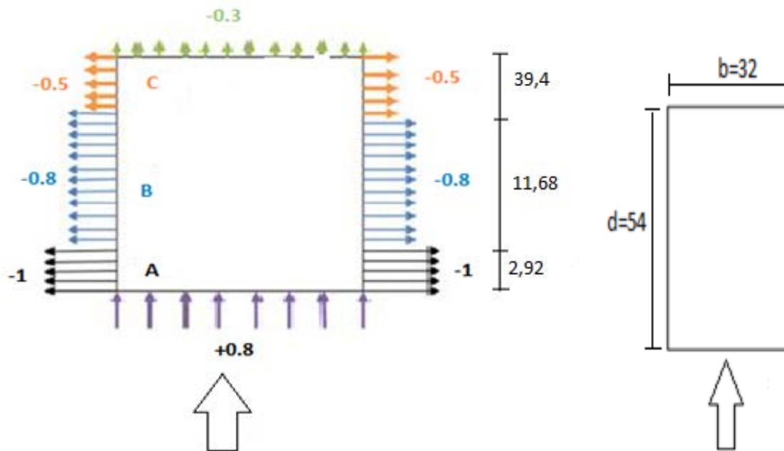
Figure II.3 Direction du vent V_3 sur les parois
