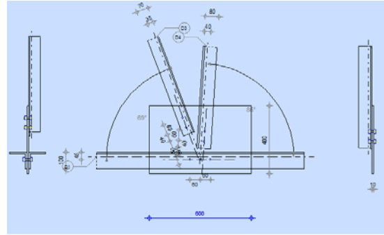
Figure VI.5 Détail d'assemblage des éléments de la ferme
