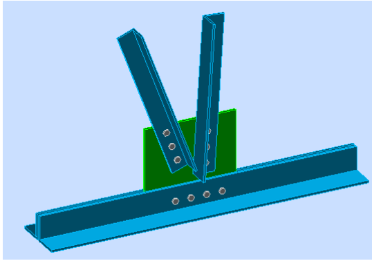
Figure VI.4 Vue en 3D de l'assemblage des éléments de la ferme
