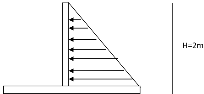
Figure VIII.3 Diagramme des poussées exercées par le remblai
