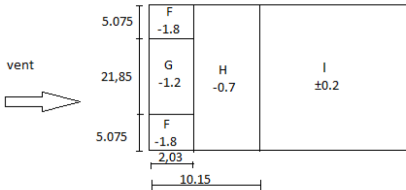
Figure II.6 Répartition des pressions sur toiture
