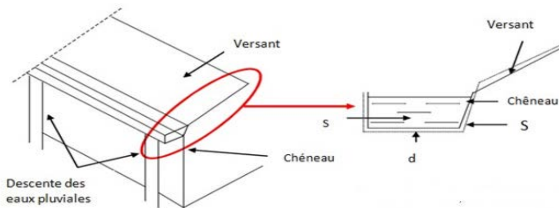
Figure III.1 Chéneau d'eau
