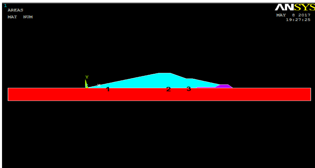
Figure III.24 : Positions pour l'analyse des paramètres Absence tapis amont
