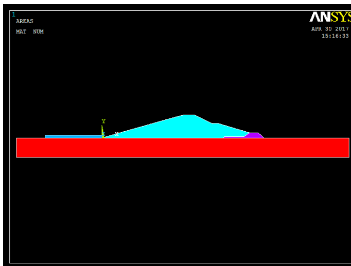
Figure III.26 : Profil géométrique Influence de la longueur de tapis amont
