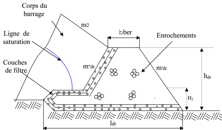
Figure II.9 : Prisme de drainage avec drain tapis interne sur fondations perméables
