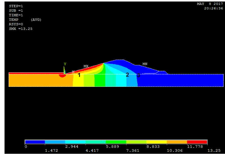
Figure III.34 : Champ de flux thermique Influence de la longueur de tapis amont L=60m
