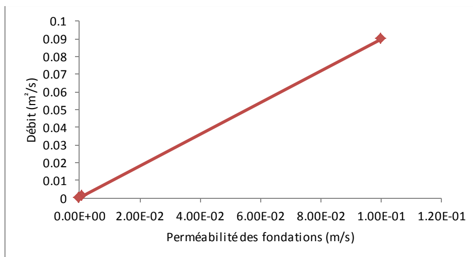
Figure III.61 : Variation des débits d'infiltration en fonction de l'influence de la perméabilité des fondations
