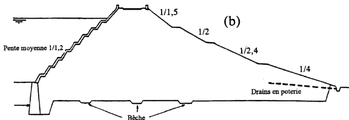
Figure I.1 : Coupes types de barrages en terre anciens (Degoutte et Gerard; 1997)
