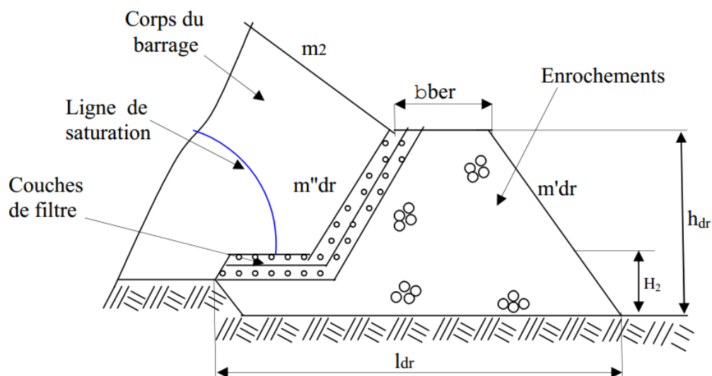
Figure II.8 : Prisme de drainage avec drain tapis interne sur fondations imperméables
