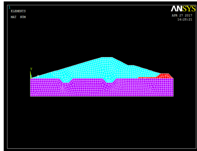
Figure III.15 : Maillage Influence des chemins d'écoulement
