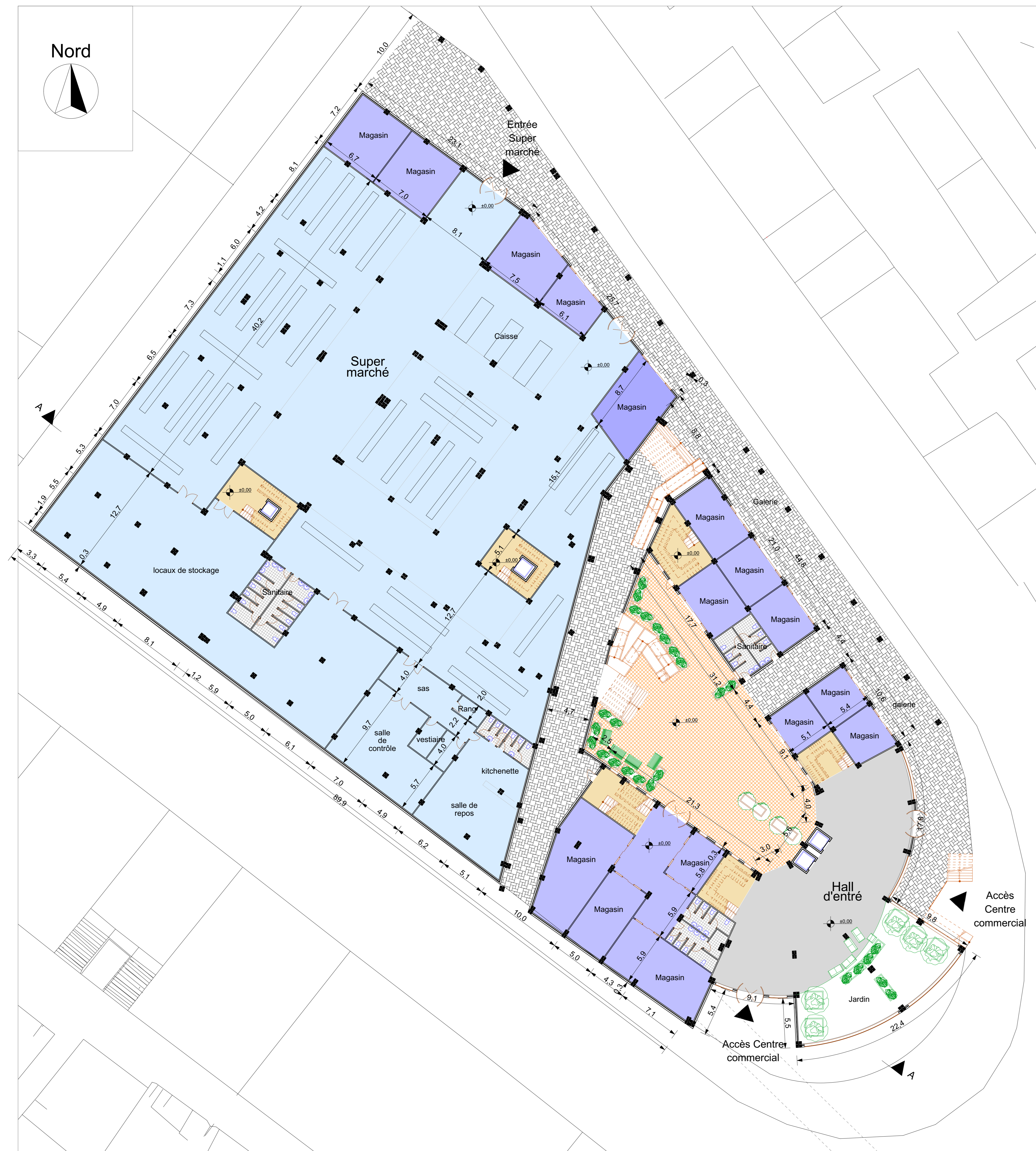
Plan de Rez de Chaussée (1ier terrain) 1/200
