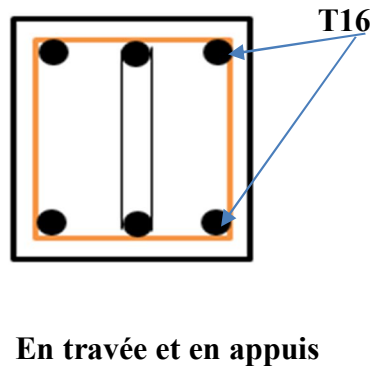
Figure VI.3: Ferraillage des poutres secondaire
