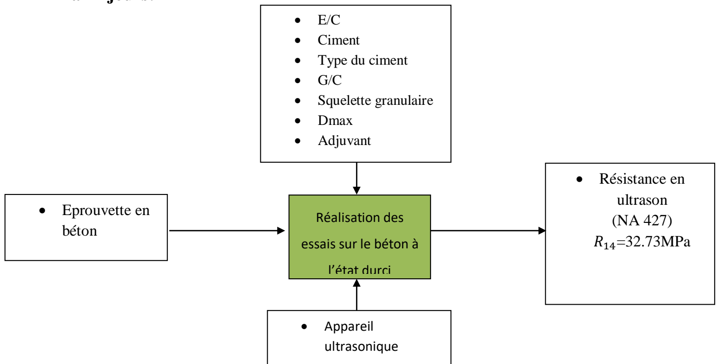
Figure 4.19 : processus d'essai d'ultrason réalisé sur le béton de la première formulation à l'état durci à 14 jours
