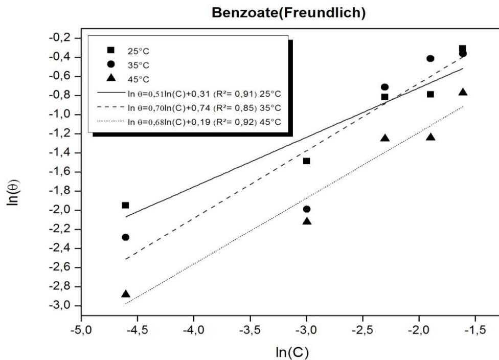
Figure 5.14 : Isothermes d’adsorption de Benzoate de sodium selon le modèle de Freundlich.
