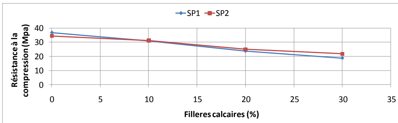
Figure IV.12 : Résistance à la compression des mortiers en fonction des taux des fillers calcaires et des superplastifiants SP1 et SP2.
