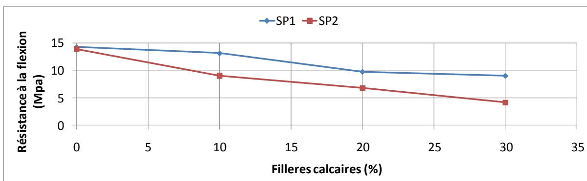
Figure IV.13 : Résistance à la flexion des mortiers en fonction des taux des fillers calcaires et des superplastifiants SP1 et SP2.
