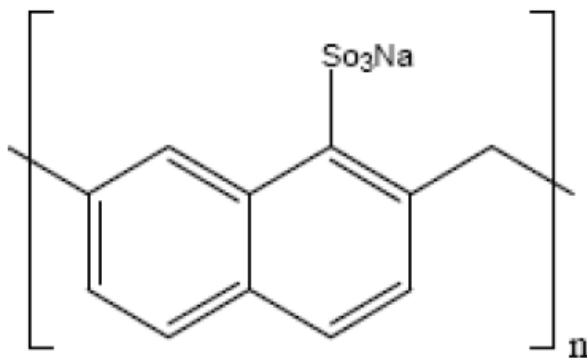
Figure II.2 : Structure chimique des polynaphtalènes sulfonates PNS
