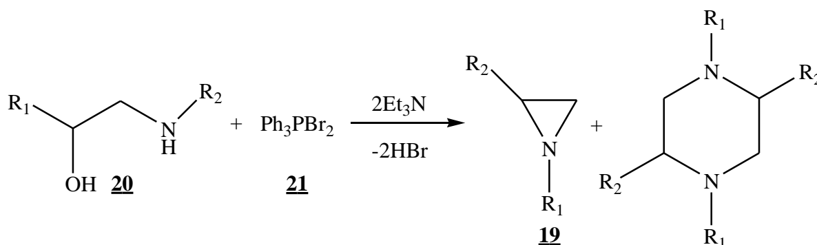
Schéma 14. Synthèse d'aziridine 19 à partir de l'α-aminoalcool 20
