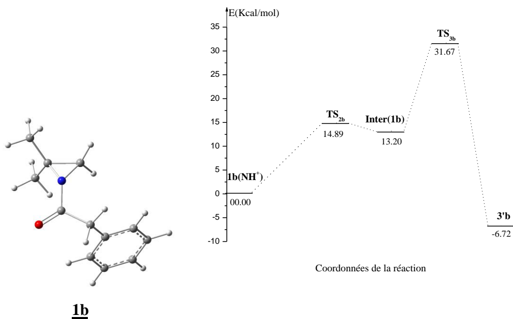
Figure 52. Profil énergétique de la rupture cyclique du 1b(NH^+) donné par la B3LYP/6-31G(d)
