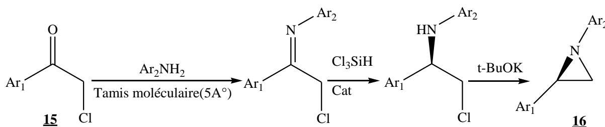
Schéma 12. Aziridination à partir d'α-chlorocétone 15
